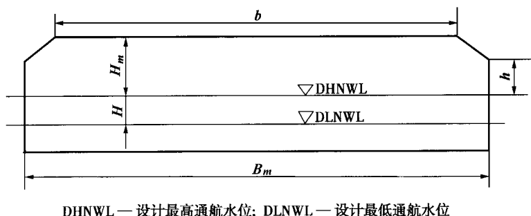
图 5-1 水上过河建筑物通航净空
