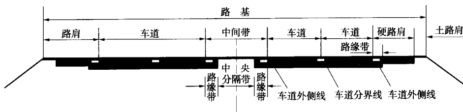
图 3-1 高速公路、一级公路路基标准横断面
