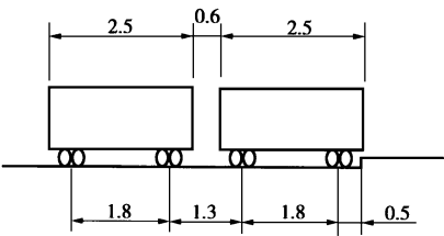
图 6.0.5 车辆荷载横向布置 (尺寸单位：m)
