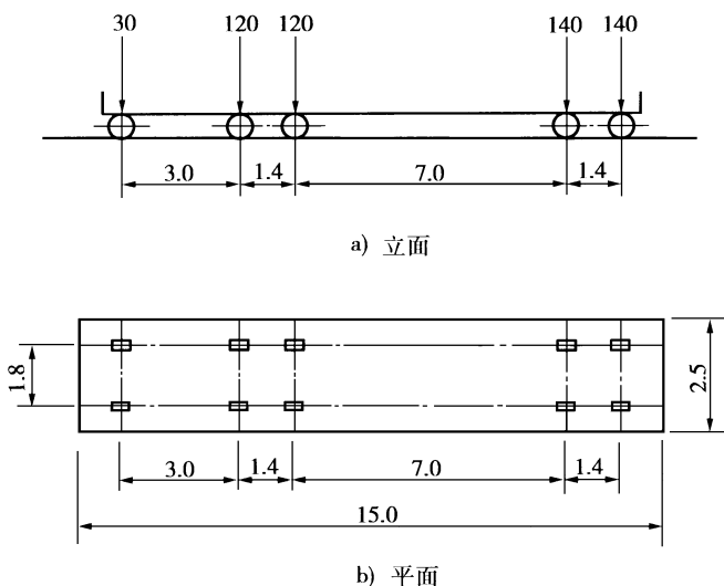
图 6.0.4 车辆荷载布置图 (轴重力单位：kN；尺寸单位：m)
