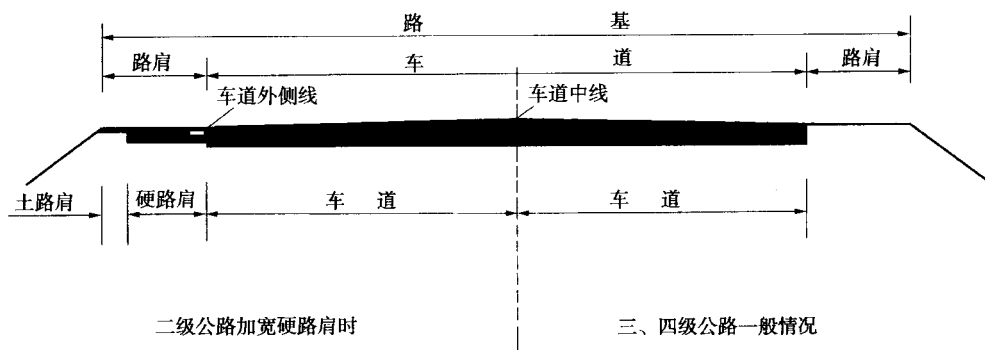
图 3-2 二、三、四级公路路基标准横断面
