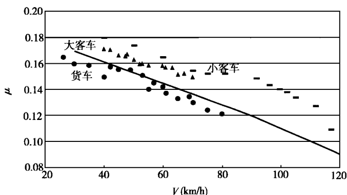
图 3-3 横向力系数取值示意图
