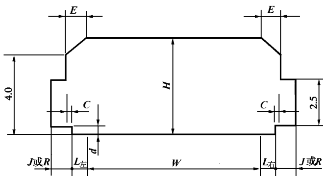
(4)隧道
