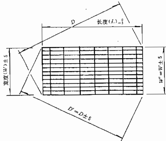
图7 钢格板对角线偏差
