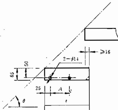
图 A2 端边板尺寸 t 及安装孔 A 的尺寸
