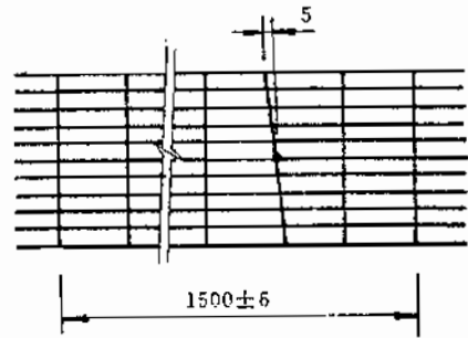
图4 横杆间距和垂直偏差
