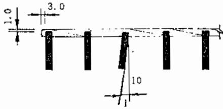
图3 负载扁钢、横杆的偏差
