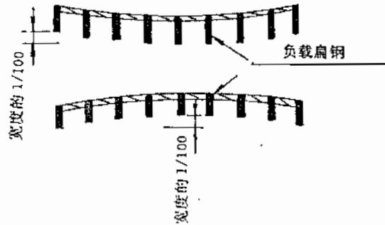
图6 横向弯曲
