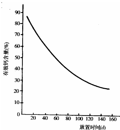
附图 4.2.2 放置时间对石灰有效钙含量的影响
