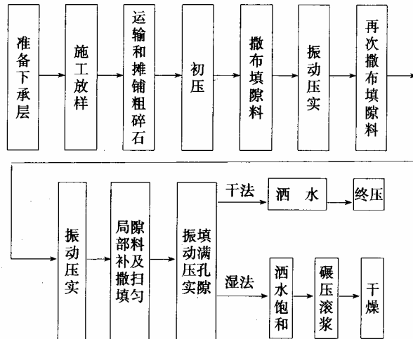
图 8.3.1 填隙碎石工艺流程图
