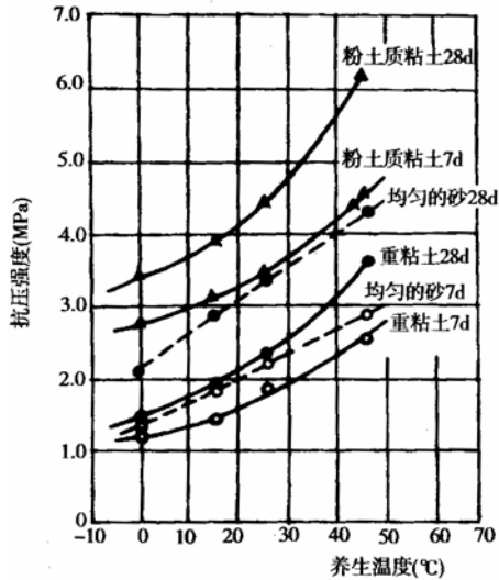
附图 3.1.5 养生温度对水泥稳定土抗压强度的影响
