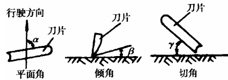
图 6.3.6 平地机刀片安装示意图
