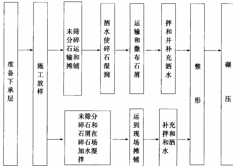
图 6.3.1 级配碎石路拌法施工工艺流程图
