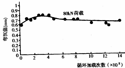
附图 6.1.5-3 级配碎石沥青表面处治弯沉演变图
