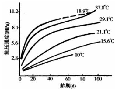
附图 5.1.5 养生温度对二灰砂砾抗压强度的影响
