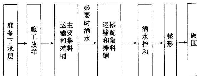
图 7.3.1 级配砾石施工工艺流程图
