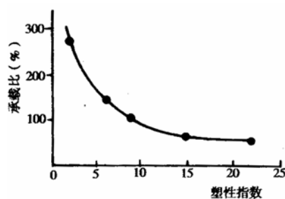
附图 6.2.5 塑性指数对级配集料承载比的影响
