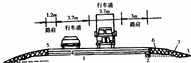
附图 6.1.5-2 路面典型横断面
