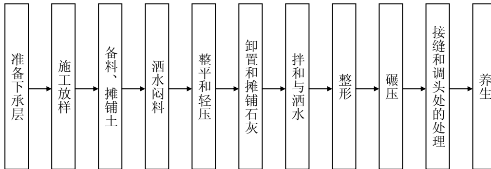
图 4.4.1 石灰稳定土路拌法施工的工艺流程
