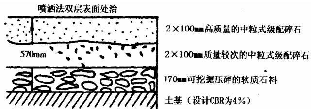
附图 6.1.5-1 维多利亚州重负荷柔性路面的典型结构
