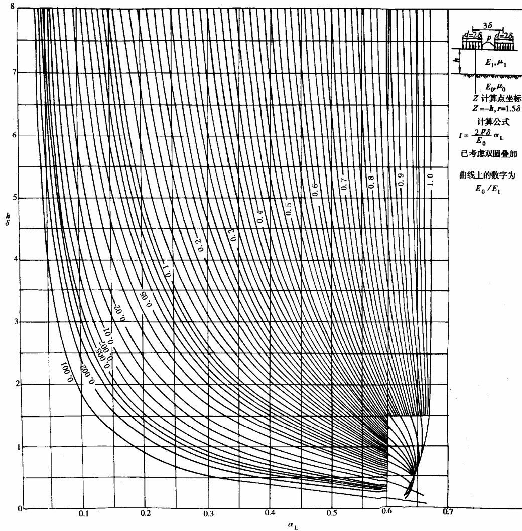
附图 A.0.3 双层体系表面弯沉系数图
