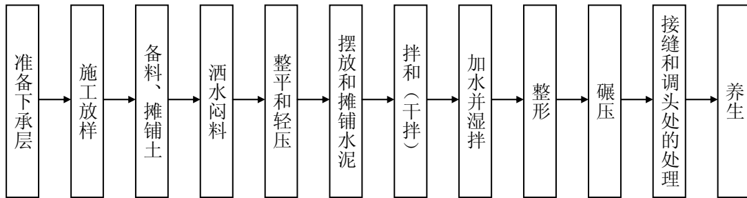
图 3.4.1 路拌法施工水泥稳定土的工艺流程
