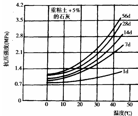
附图 4.1.5 养生温度对石灰稳定土抗压强度的影响
