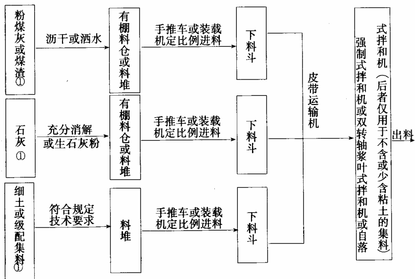
图 5.5.2 石灰工业废渣稳定土的集中拌和工艺流程 ②
