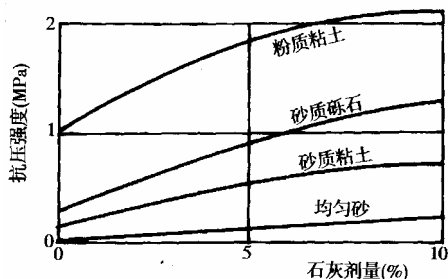
附图 4.2.1 土质对石灰稳定土抗压强度的影响
