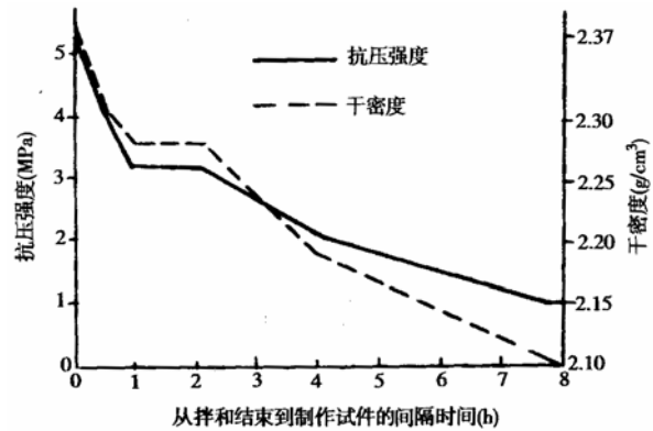
附图 3.1.7 延迟时间对水泥砂砾的强度和干密度的影响
