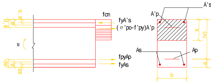
图 5.1.3 矩形截面受弯构件正截面受弯承载力计算
