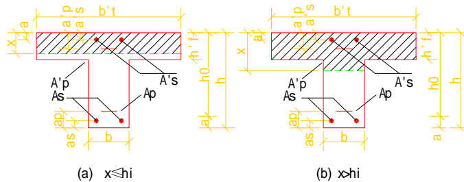
图 5.1.4 T 形截面受弯构件受压区高度位置
