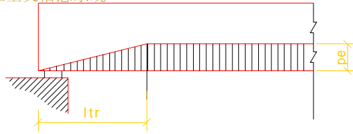
图 A.0.2 预应力冷轧带肋钢筋的预应力传递长度 l_{tr} 范围内有效预应力值变化 预应力冷轧带肋钢筋的预应力传递长度 l_{tr} (mm) 表 A.0.2
