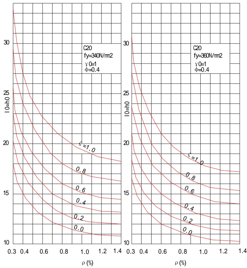
图 C.0.1 冷轧带肋钢筋混凝土受弯构件 不需作挠度验算的最大跨高比
