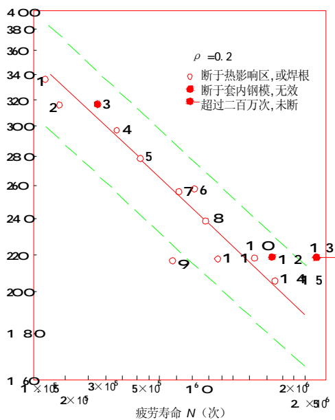
图 6.0.12 钢筋焊接接头疲劳试验 S-N 曲线
