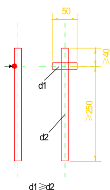
图 3.0.1-1 钢筋焊接 骨架试样
