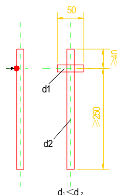
图 3.0.1-2 钢筋焊接 网试样
