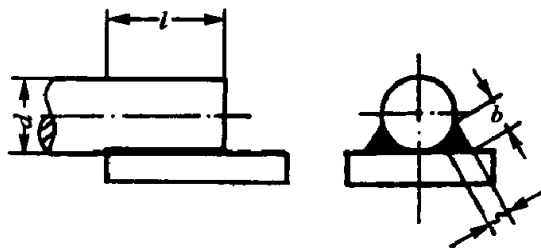
图 4.4.9 钢筋与钢板搭接焊接头
