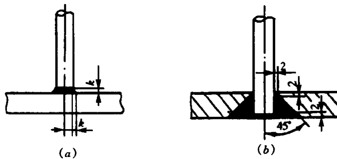
图 4.4.8 预埋件钢筋电弧焊 T 型接头
