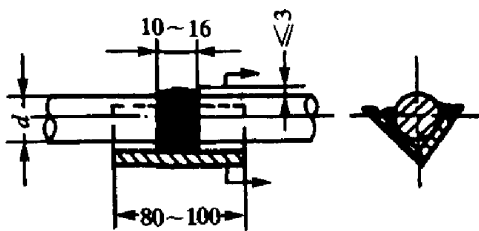
图 4.4.6 钢筋熔槽帮条焊接头
