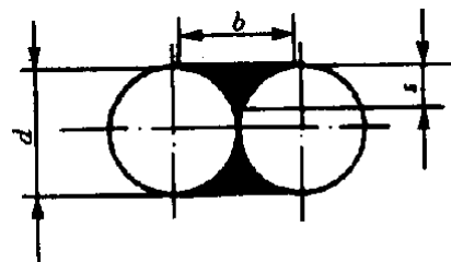
图 4.4.4 焊缝尺寸示意图
