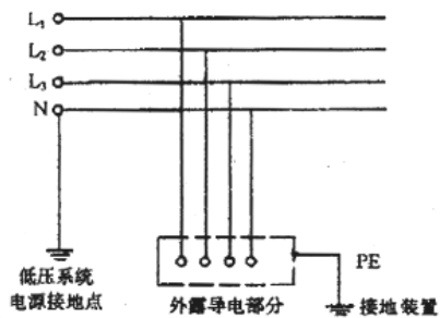
图 C.1-4 TT 系统
