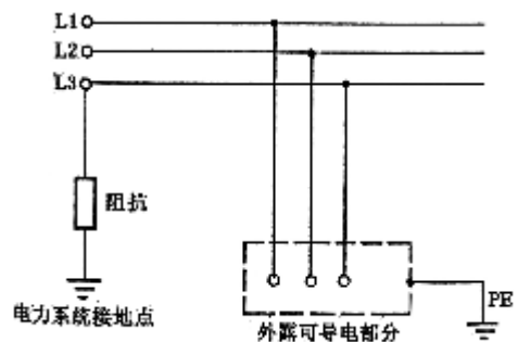
图 C.1-5 IT 系统
