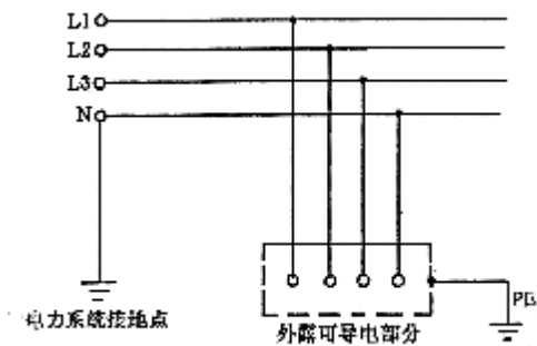
图 C.1-4 TT 系统
