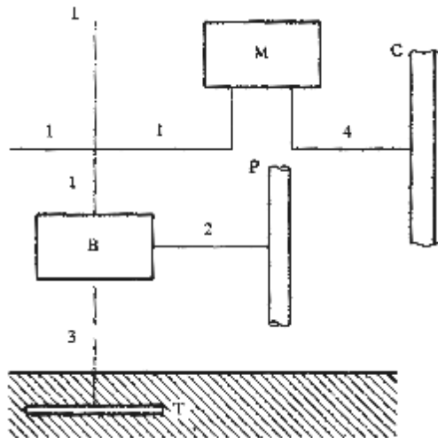
图 12.3.5 等电位联结
