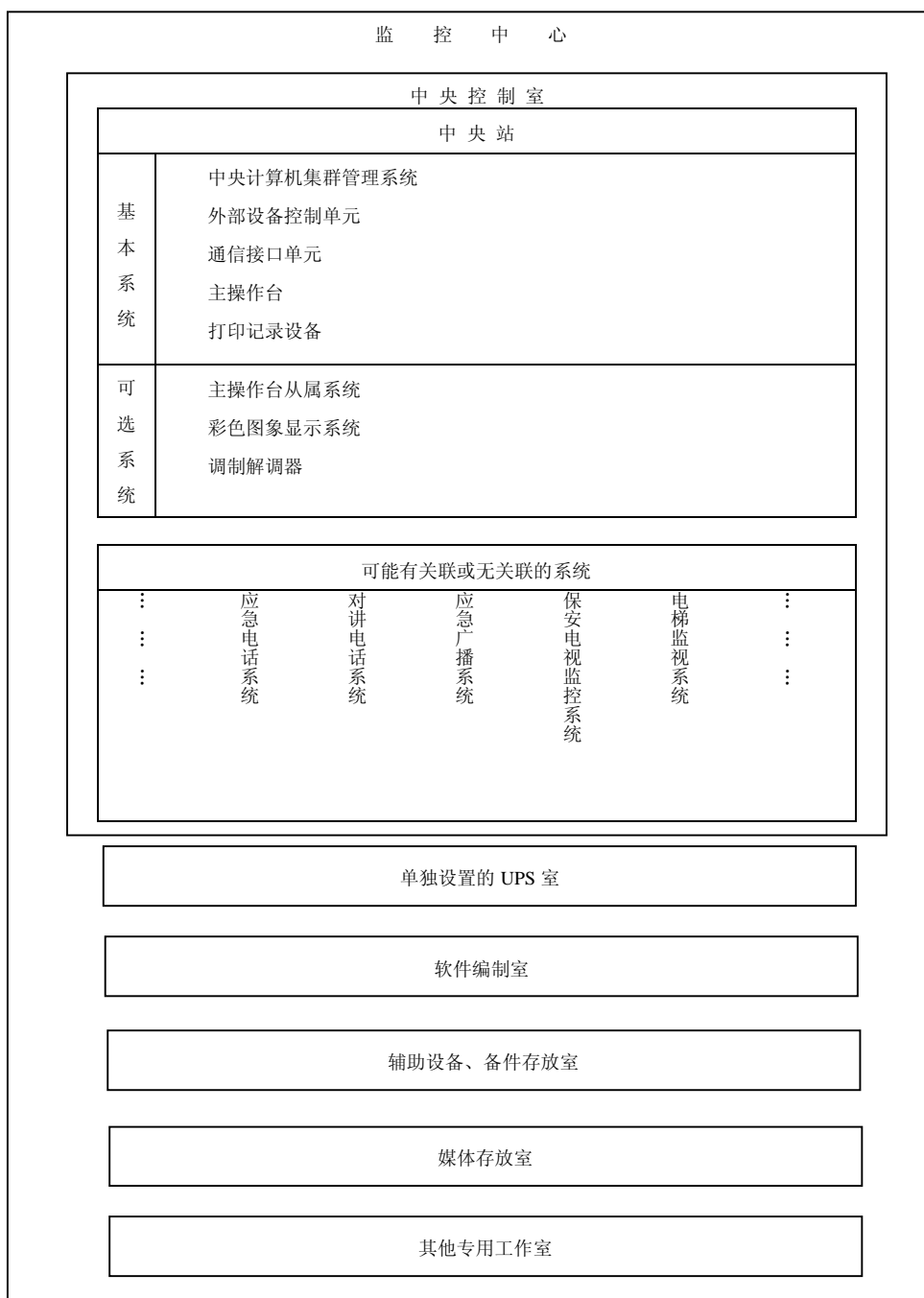
图 18.2.12 中央站——中央控制室——监控中心的组态
