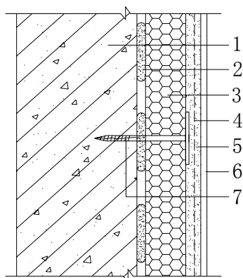
图 6.1.1 EPS 板薄抹灰系统
