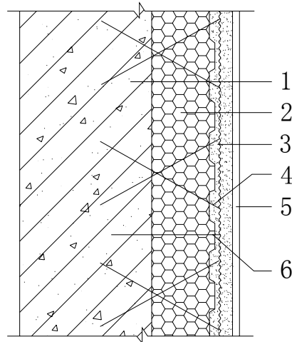
图 6.4.1 有网现浇系统
