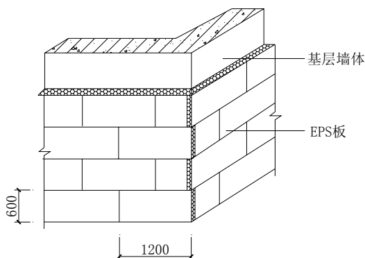
图 6.1.9-1 EPS 板排板图
