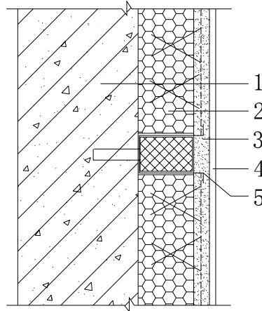
图 6.5.1 机械固定系统
