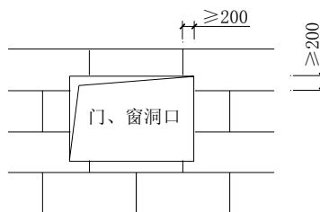
图 6.1.9-2 门窗洞口 EPS 板排列
