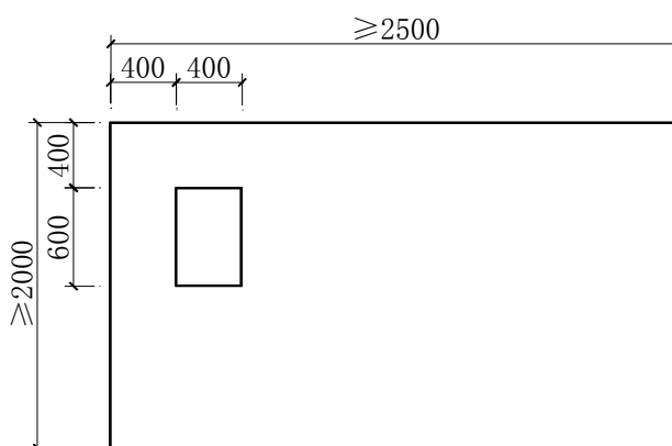
图 A.2.1 试样
