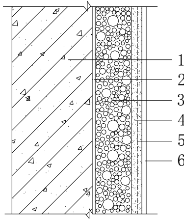
图 6.2.1 保温浆料系统
