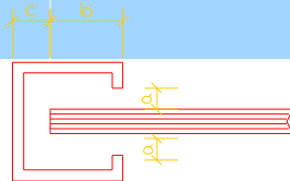
图 6.2.5-1 玻璃与槽口的配合
