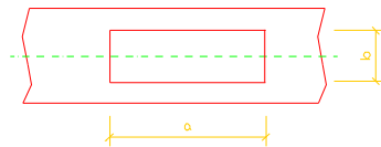
图 6.2.2-1 铣槽位置
