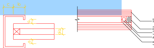
图 6.2.5-2 中空玻璃与槽口的配合
