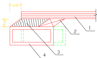
图 5.6.6 结构硅酮密封胶粘结厚度
