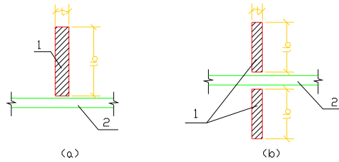
图 5.5.8 全玻璃幕墙玻璃肋截面尺寸 (a) 单肋; (b) 双肋 1—玻璃肋; 2—幕墙玻璃
