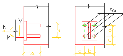
图 5.7.10 由锚板和直锚筋组成的预埋件
