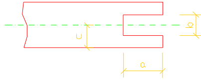
图 6.2.2-2 铣豁位置
