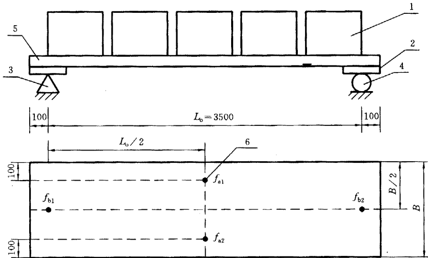
1—加载法码；2—承压板（宽 100mm，厚 6~15mm 的钢板）；3—固定铰支座； 4—滚动铰支座；5—试件；6—百分表 f_{a1} 、 f_{a2} 、 f_{b1} 、 f_{b2} 。
