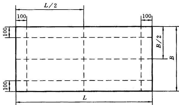
图 1 长度、宽度的测量位置
