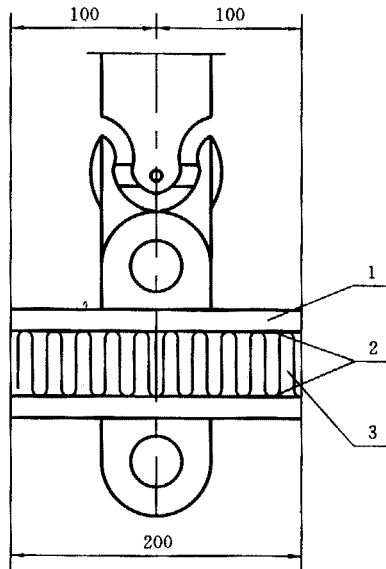
1—平钢板; 2—粘结剂接合处; 3—试件
