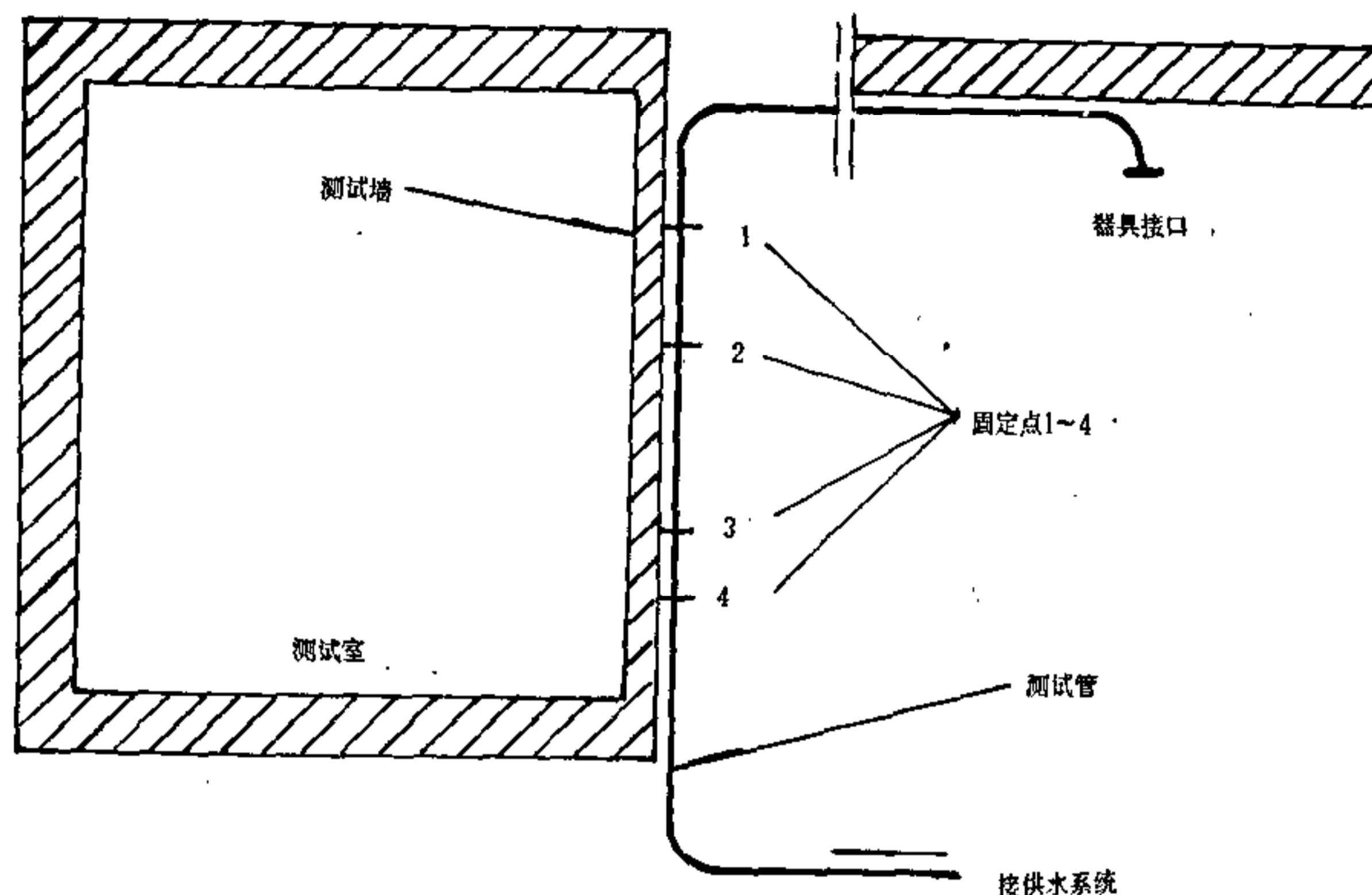
图 I1 测试布置示例
