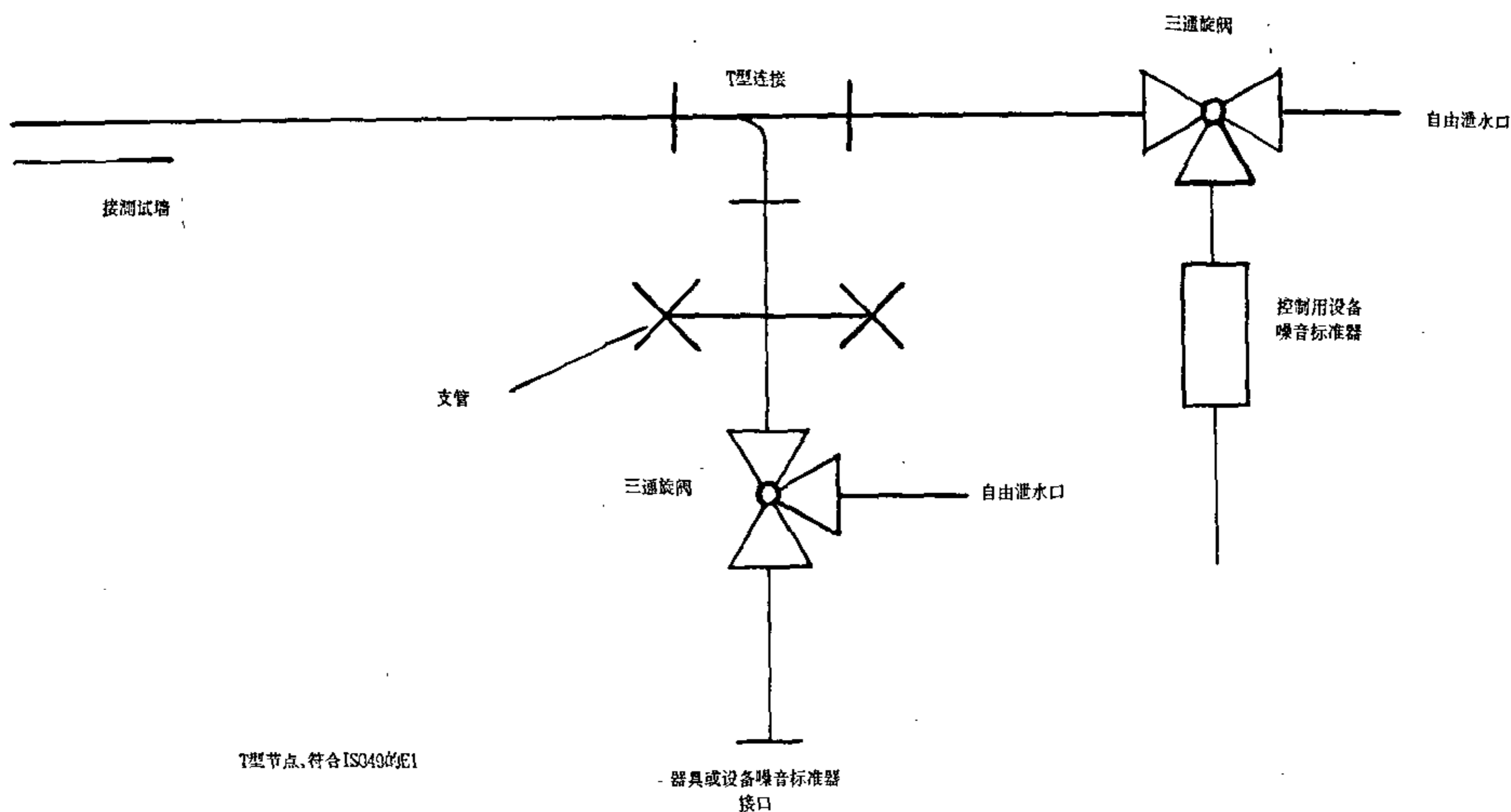
图 12 设备的安装和试验布置校对示例
