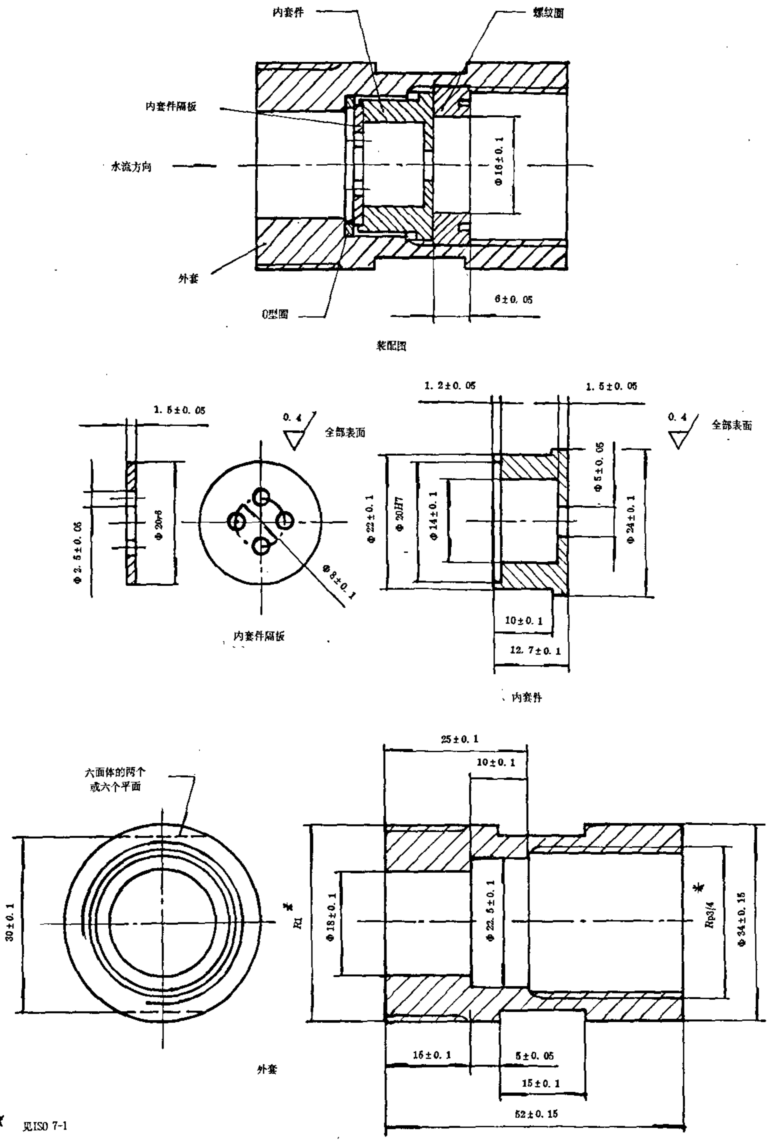
图13 设备噪音标准器
