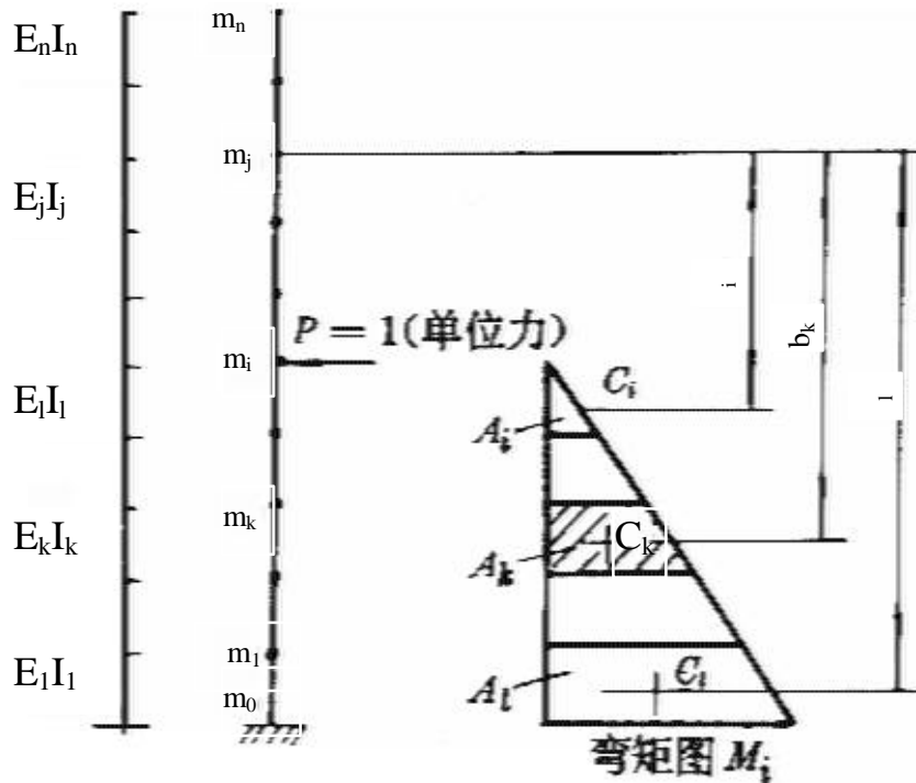
图 A2 位移计算图
