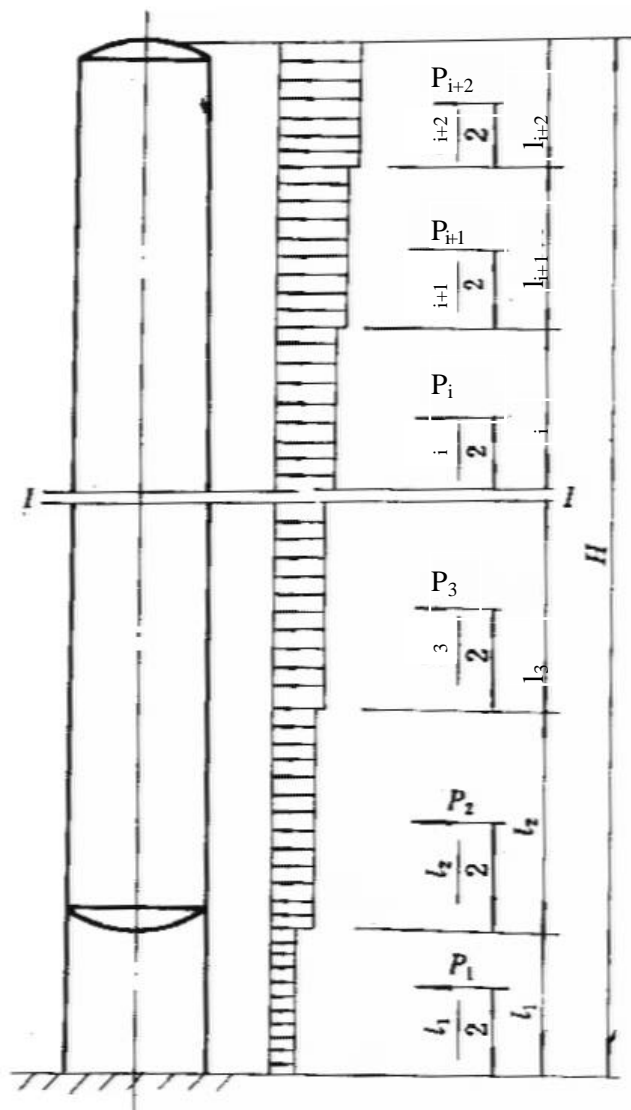
图 6-6 风弯矩计算简图
