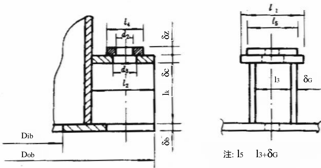
图 6-11 地脚螺栓座尺寸
