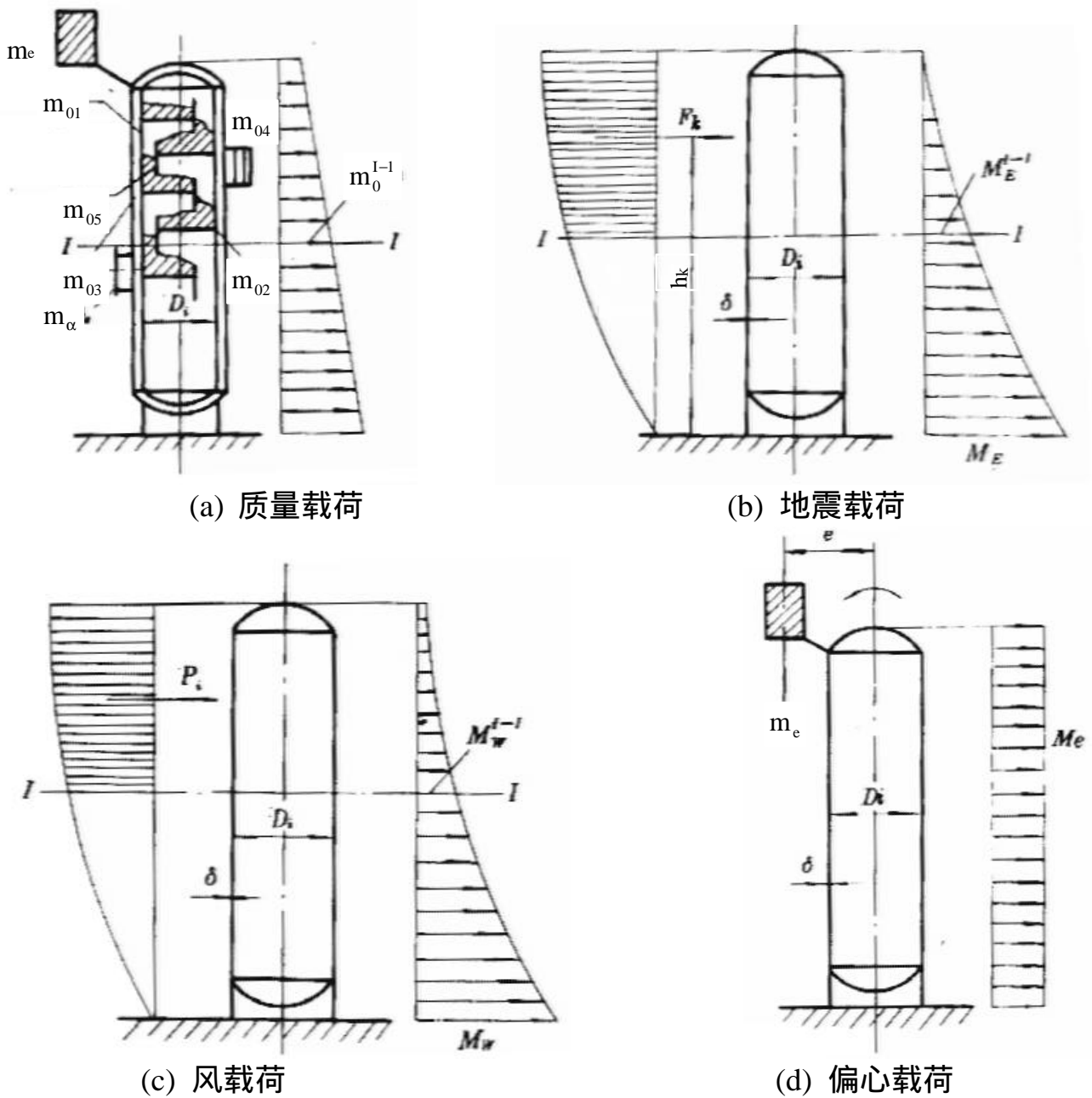
图 6-1 塔器各种载荷示意图
