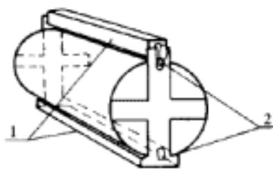
图 D.0.4-2 定位架
