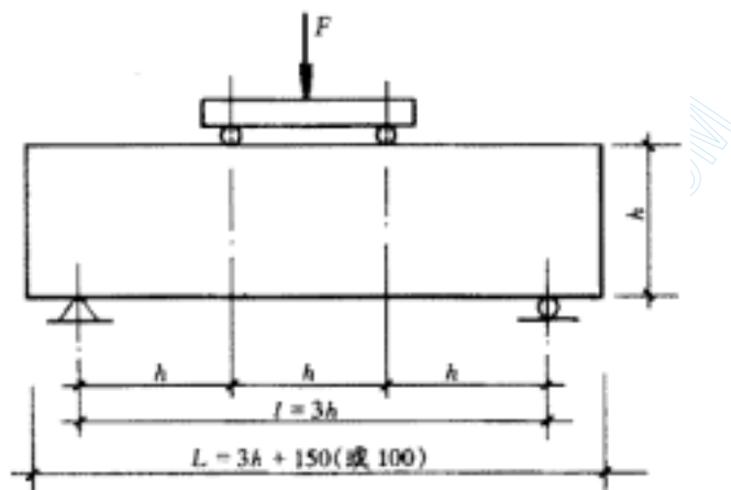
图 10.0.3 抗折试验装置
