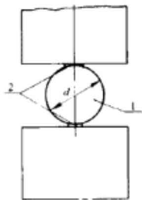
图 D.0.4-1 劈裂抗拉试验
