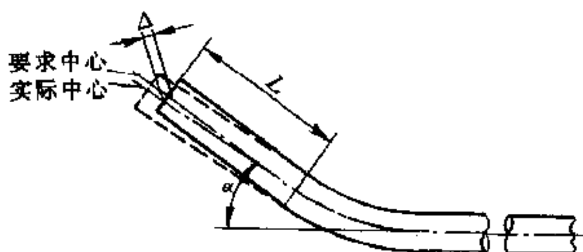
图 4.2.8 弯曲角度及管端中心偏差
