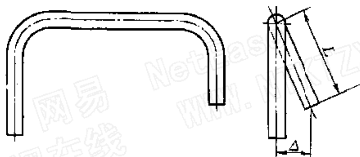
图 4.2.9 U形弯管平面度
