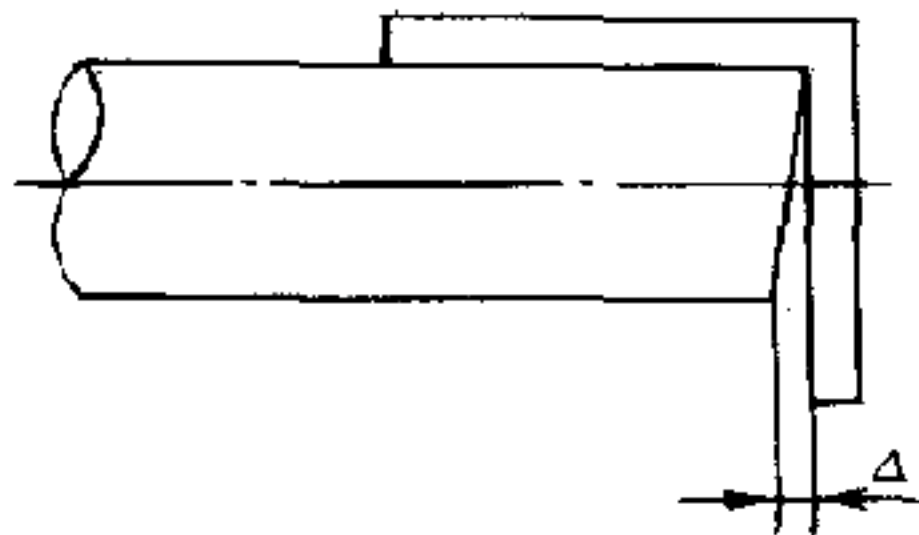
图 4.1.5 管子切口端面倾斜偏差
