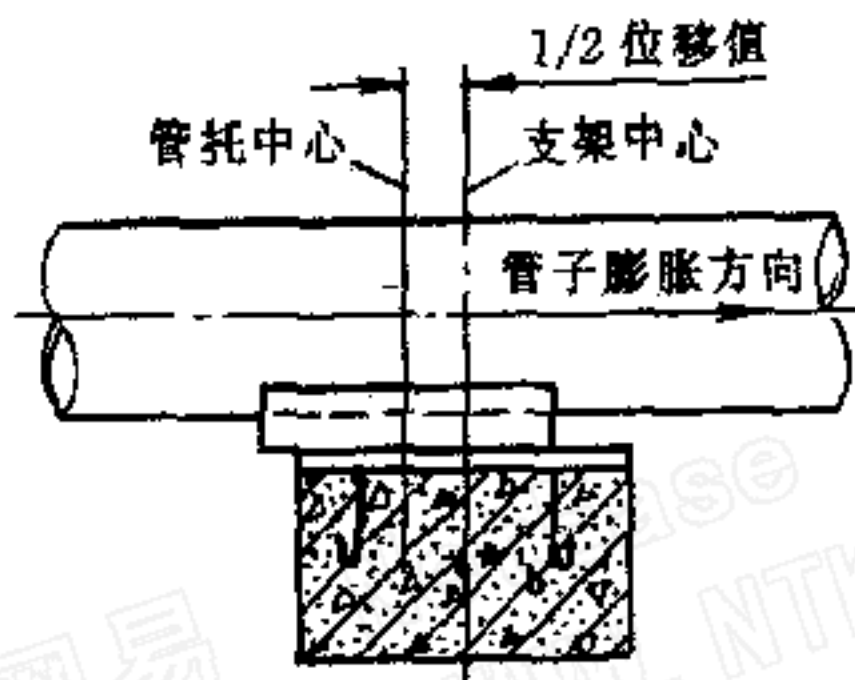
图 6.11.4 滑动支架安装位置
