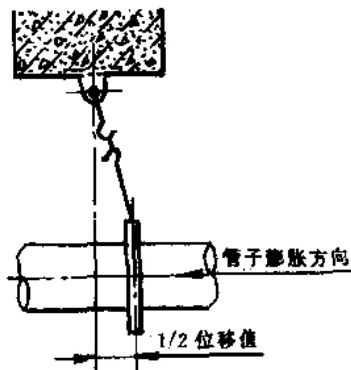
图 6.11.2 有热位移管吊架安装
