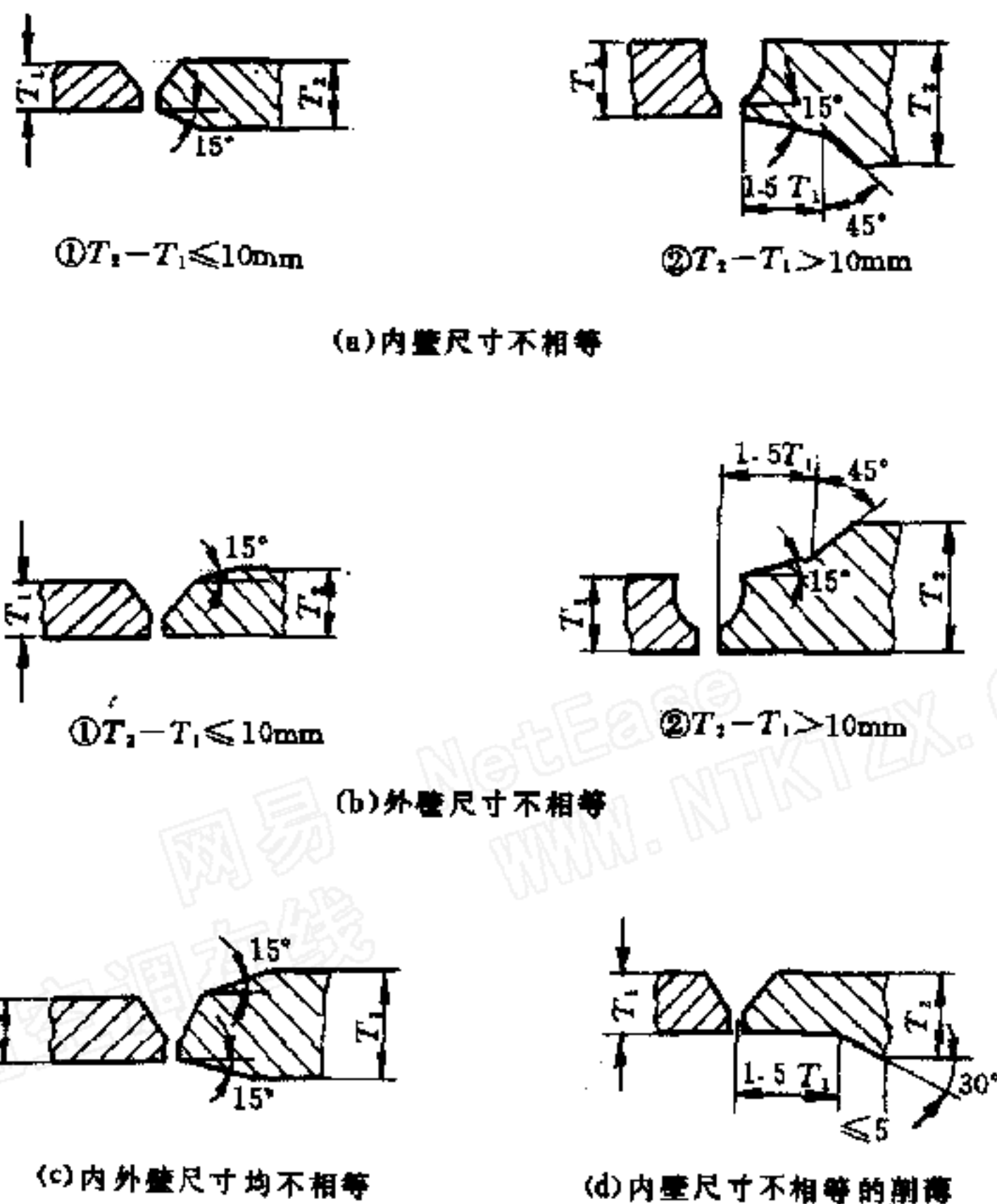
图 5.0.8 焊件坡口形式
