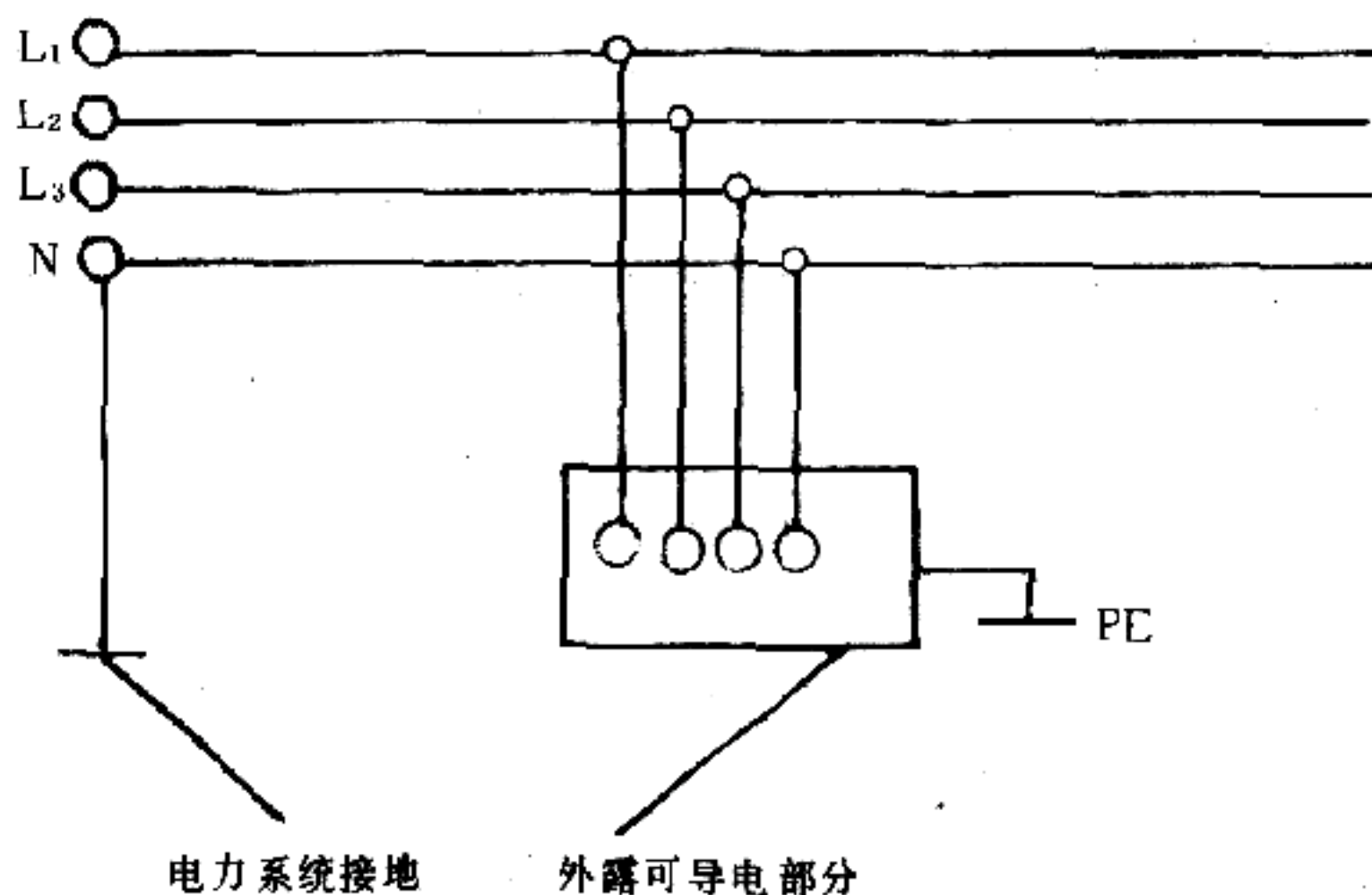
图 4.1.1-2 TT 系统
