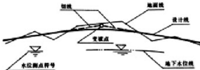
图 3.2.2 道路设计线、原地面线、地下水位线的标注
