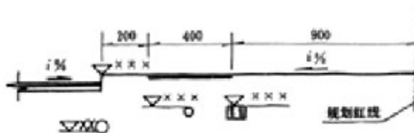
图 3.3.3 横断面图中管涵、管线的标注
