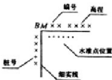
图 3.2.6 水准点的标注
