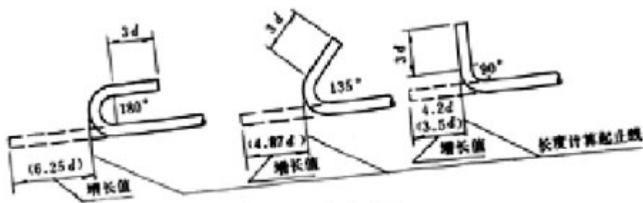
图 4.2.5 标准弯钩
