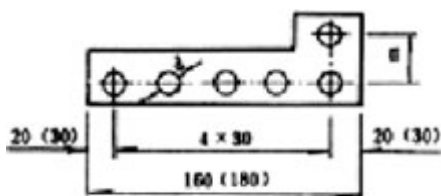
图 2.7.11 相似图形的标注
