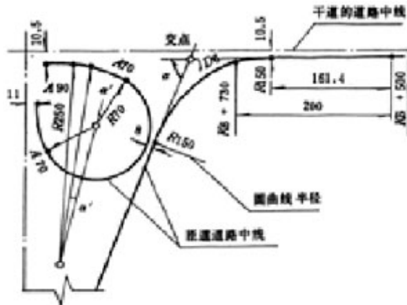
图 3.4.6 立交工程线形布置图
