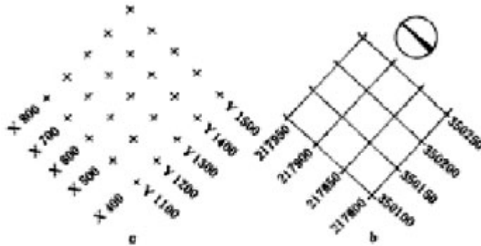
图 2.5.1 坐标网格及标线
