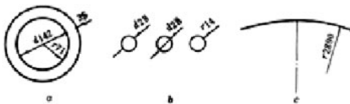
图 2.7.8 半径与直径的标注
