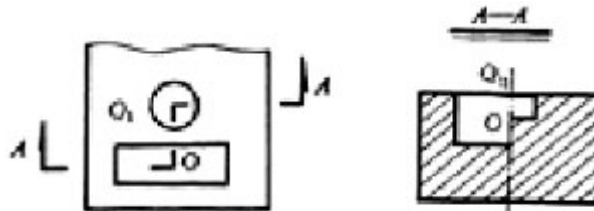
图 2.8.4 阶梯剖的标注
