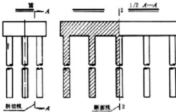
图 2.8.3 视图的剖切及标注
