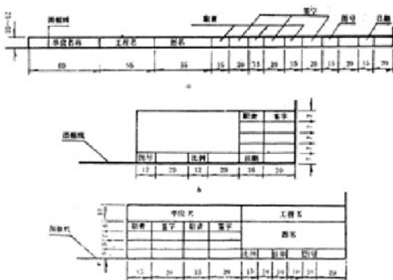
图 2.2.2 图 标(单位:mm)
