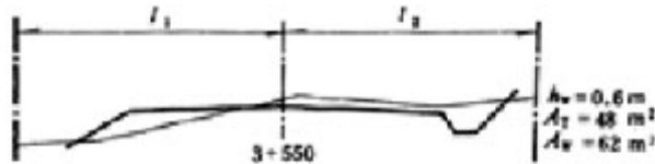
图 3.3.5 横断面图中填挖方的标注
