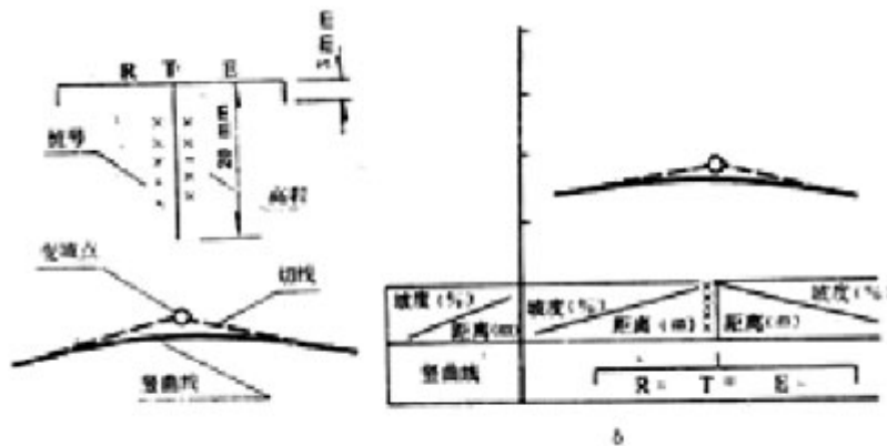
图 3.2.4 竖曲线的标注
