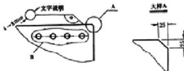
图 2.7.6 大样图范围的标注
