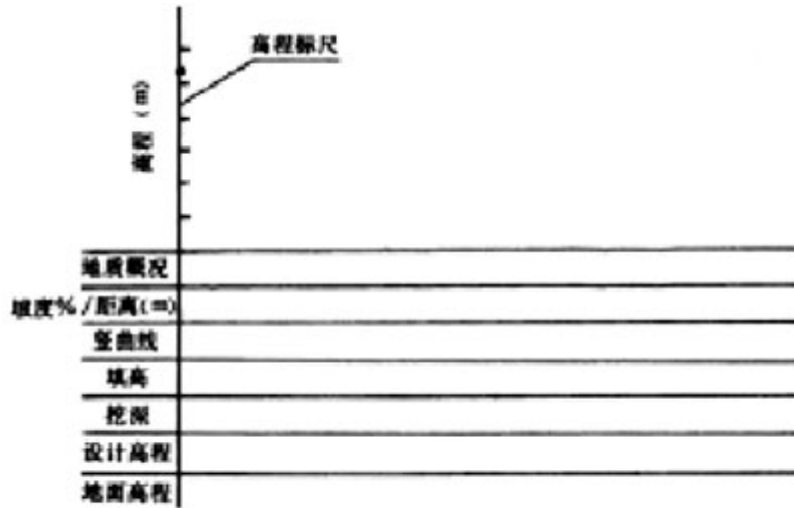
图 3.2.1 纵断面图的布置
