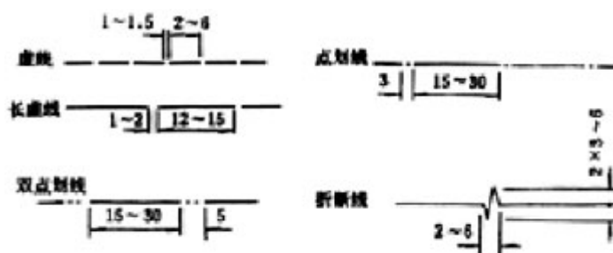
图 2.4.4 图线的画法(单位:mm)
