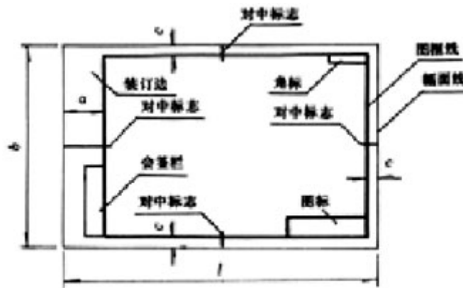
图 2.1.1 幅面格式
