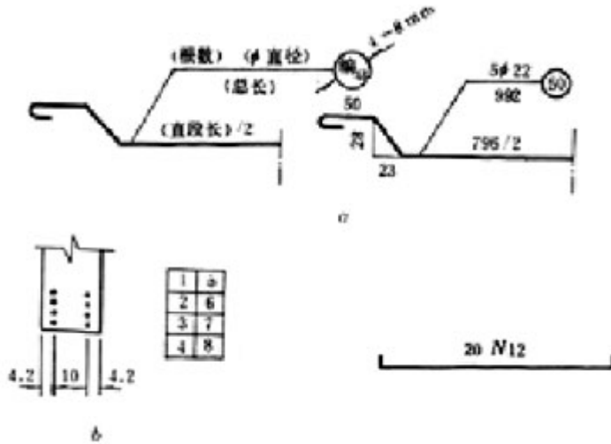
图 4.2.3 钢筋的标注
