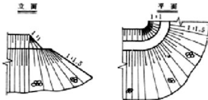
图 4.1.2 边坡和锥坡的标注
