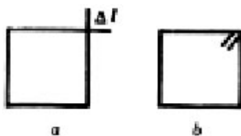
图 4.2.8 箍筋大样
