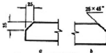
图 2.7.12 倒角的标注
