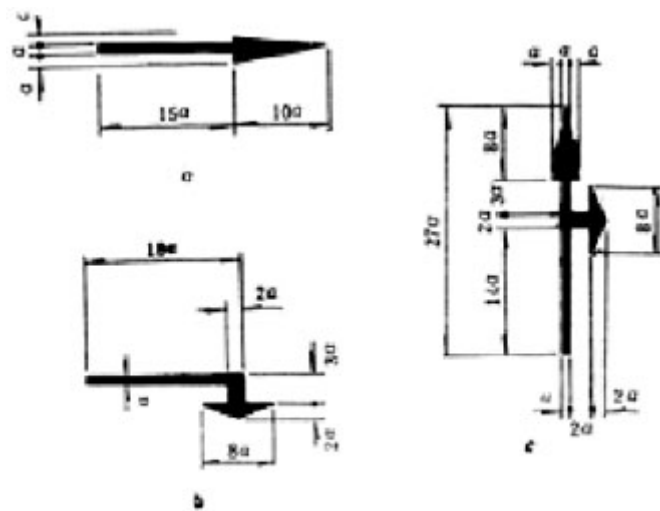
图 5.1.12 车流向标线
