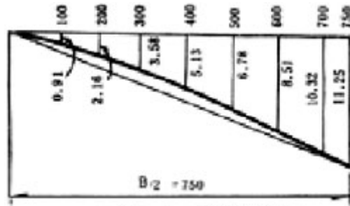
图 3.3.8 路拱曲线大样
