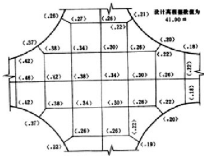
图 3.4.3 水泥混凝土路面高程标注
