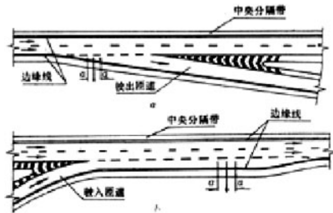
图 5.1.10 匝道出口、入口标线
