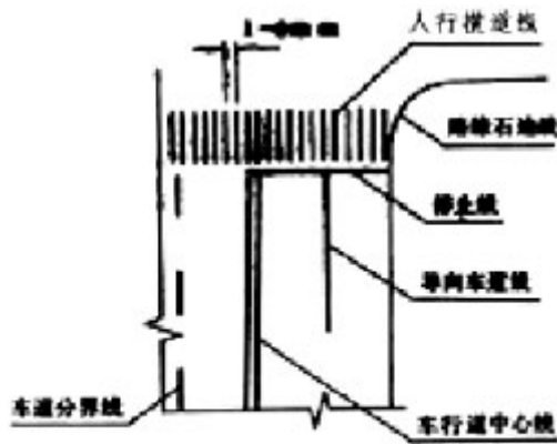
图 5.1.5 停止线位置
