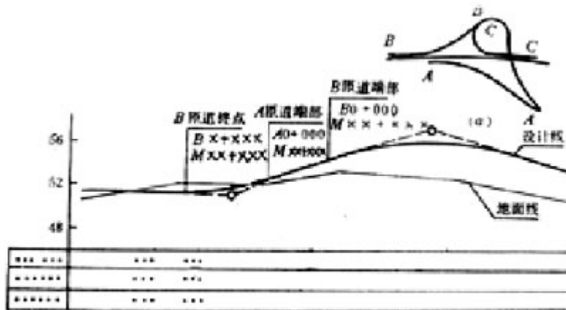
图 3.4.7 互通立交纵断面图匝道及线形示意
