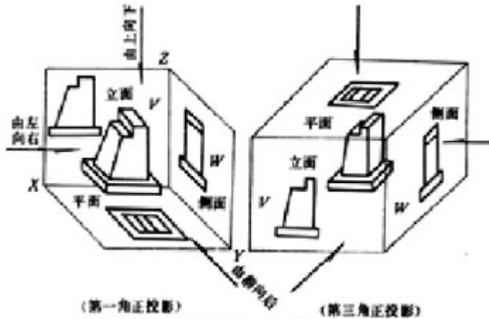
图 2.8.1 物体的投影
