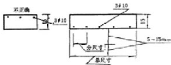
图 2.7.4 尺寸线的标注
