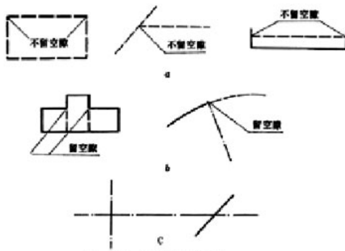
图 2.4.5 图线相交的画法
