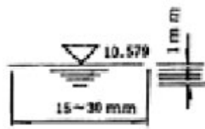
图 2.7.15 水位的标注
