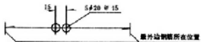
图 4.2.10 钢筋的简化标注
