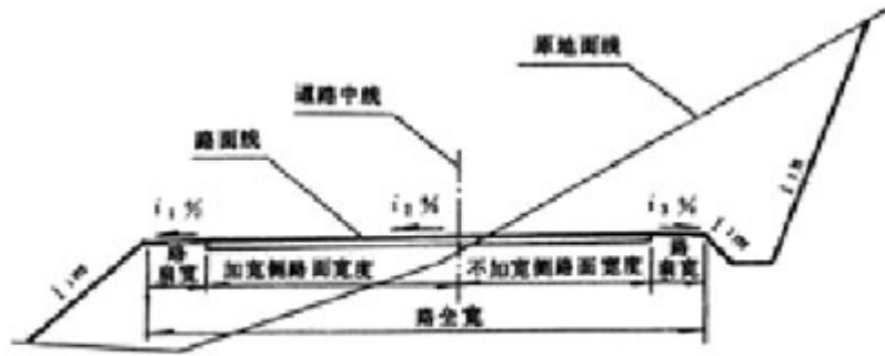
图 3.3.4 道路超高、加宽的标注
