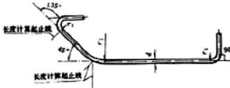
附图 1.1 钢筋的标准弯折示意图
