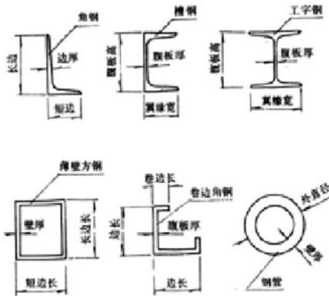
图 4.4.3 型钢各部位名称
