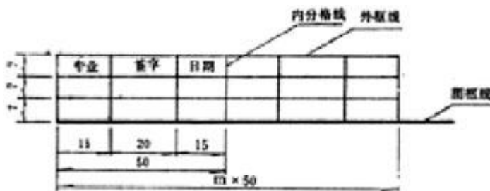
图 2.2.3 会签栏(单位:mm)
