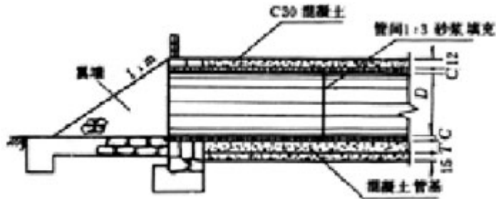
图 4.1.1 砖石、混凝土结构的材料标注
