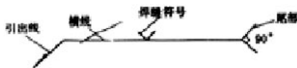
图 4.4.6—1 焊缝的标注法
