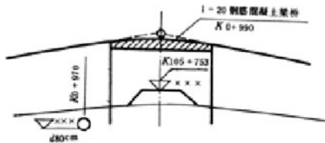
图 3.4.8 简单立交中低位道路及构造物标注
