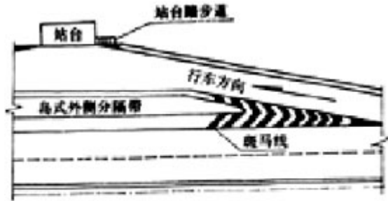
图 5.2.1 交通岛标志
