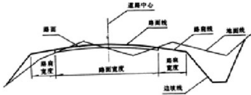
图 3.3.1 横断面图
