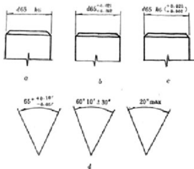
图 4.4.10 公差标注
