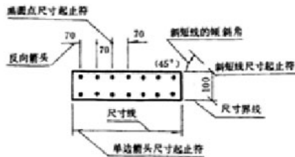
图 2.7.2 尺寸要素的标注
