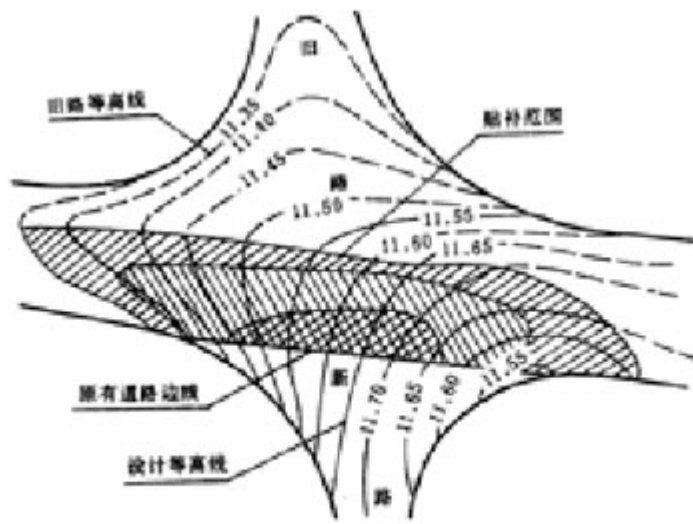
图 3.4.2 新旧路面的衔接
