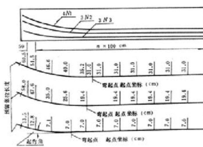
图 4.3.5 预应力钢筋大样
