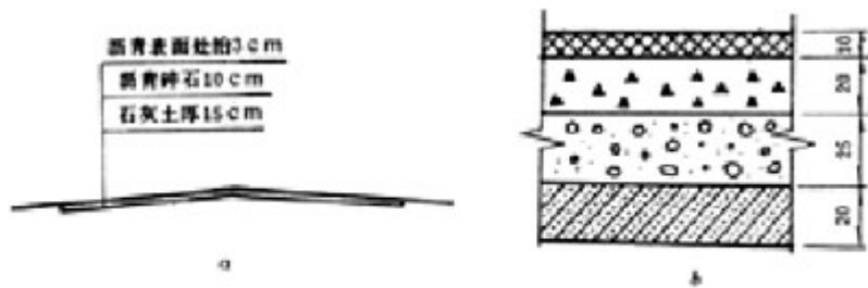
图 3.3.7 路面结构的标注
