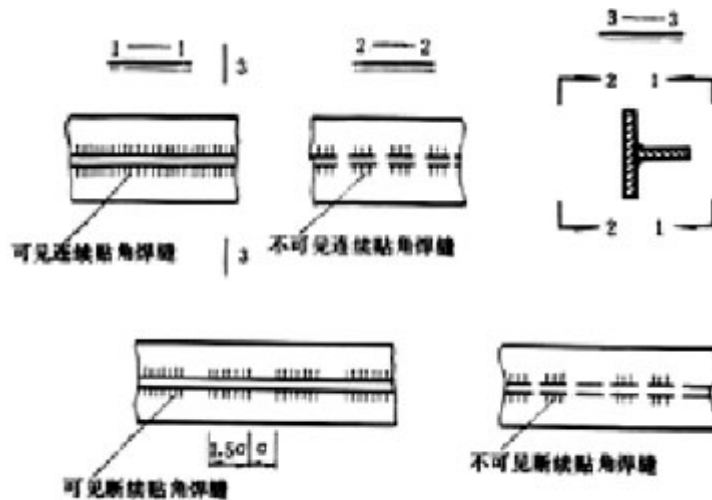
图 4.4.6—2 焊缝的图示法
