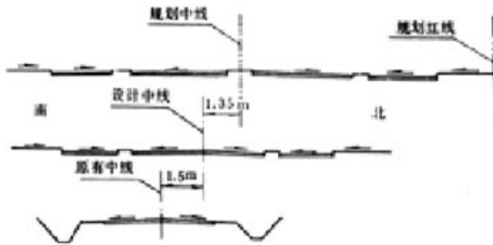
图 3.3.2 不同设计阶段横断面
