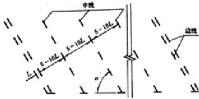
图 5.1.9 停车位标线
