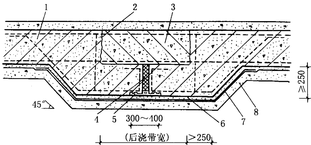
图 5.2.3 后浇带超前止水构造
