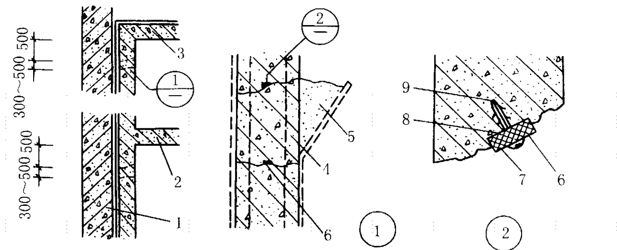
图 8.4.2 逆筑法施工接缝防水构造
