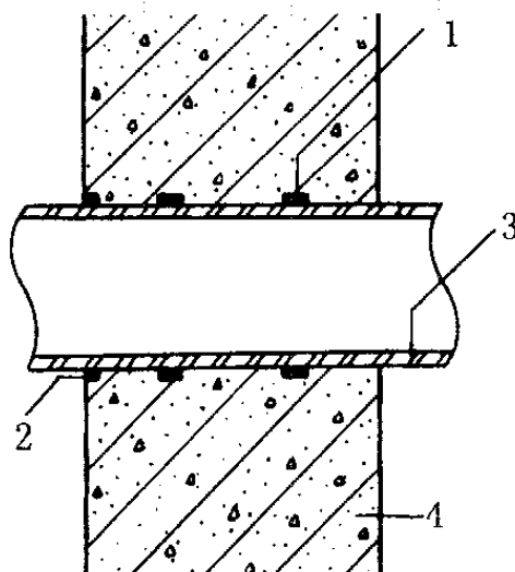
图 5.3.3-2 固定式穿墙管防水构造(二)
