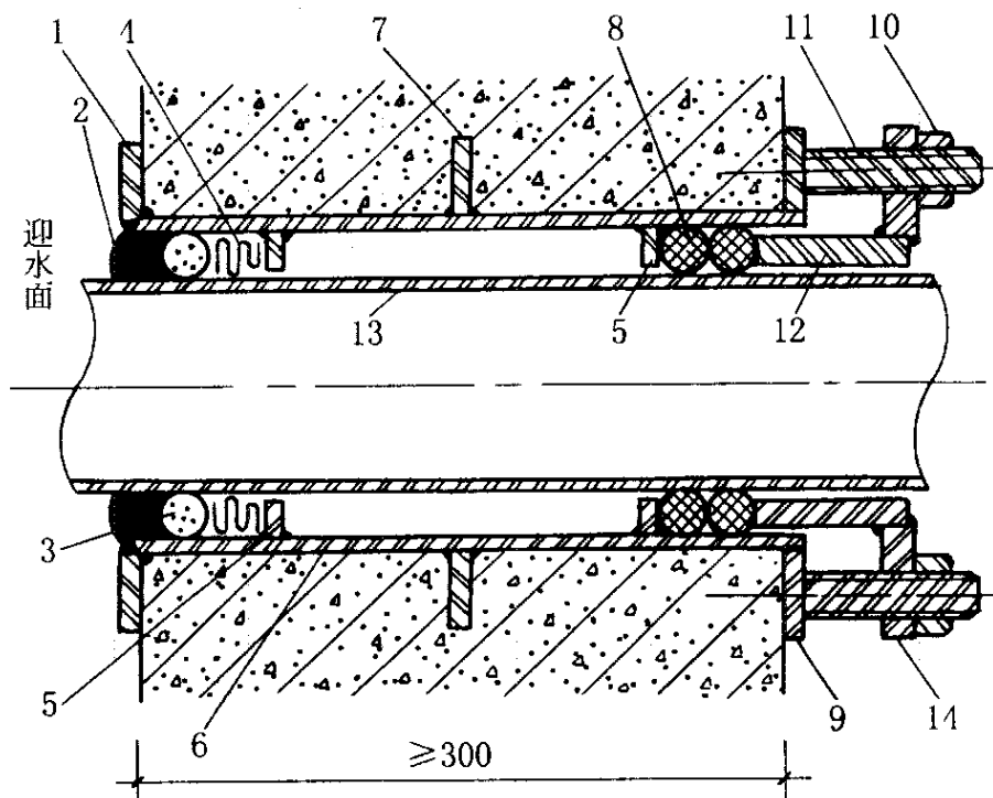
图 5.3.4 套管式穿墙管防水构造
