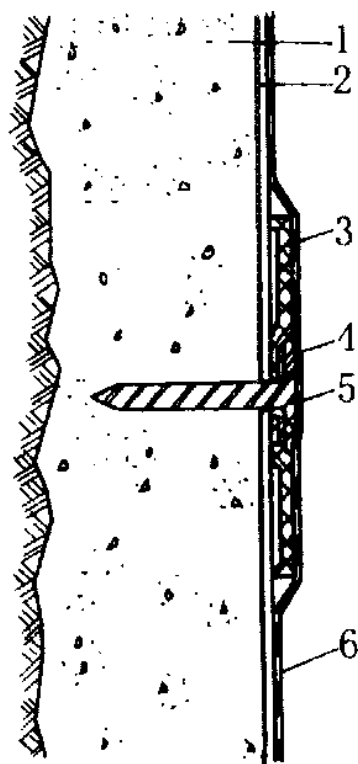
图 4.5.5 暗钉圈固定缓冲层示意图
