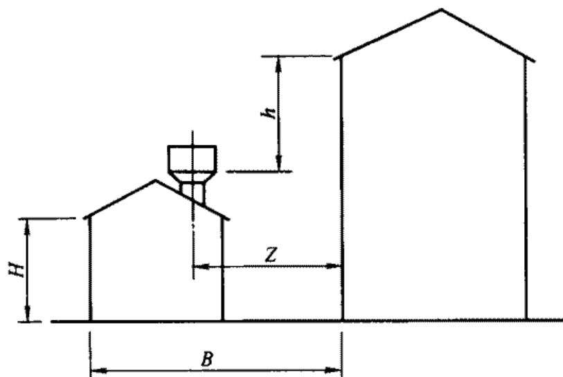
图 5.2.10-2 风帽与建筑物的相关尺寸
