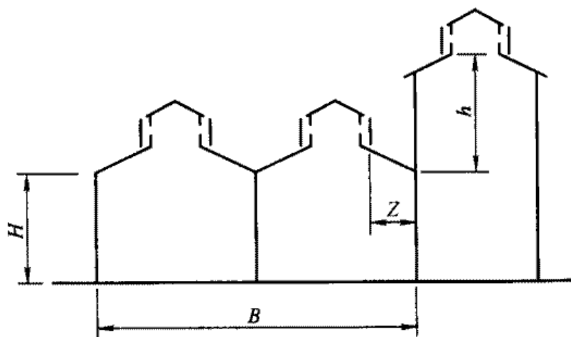
图 5.2.10-1 避风天窗与建筑的相关尺寸
