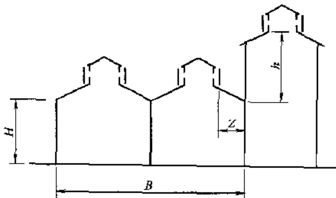
图 5.2.10-1 避风天窗与建筑的相关尺寸
