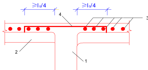
图 10.1.6 现浇板中与梁垂直的构造钢筋
