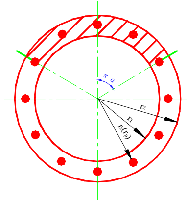
图 7.3.7 沿周边均匀配筋的环形截面
