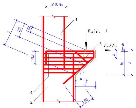
图 10.8.1 牛腿的外形及钢筋配置
