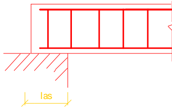
图 10.2.2 纵向受力钢筋伸入梁筒支支座的锚固
