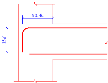
图 10.4.1 梁上部纵向钢筋 在框架中间层端节点内的锚固
