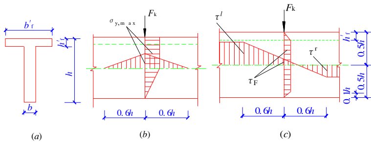
图 8.1.7 预应力混凝土吊车梁集中力作用点附近的应力分布 (a) 截面；(b) 竖向压应力 \sigma_y 分布；(c) 剪应力 \tau 分布
