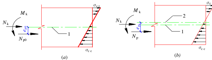
图 6.1.11 预应力混凝土构件施工阶段验算
