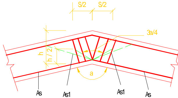
图 10.2.14 钢筋混凝土梁内折角处配筋
