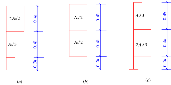
图 10.7.9-3 连续深梁中间支座截面纵向受拉钢筋在不同高度范围内的分配比例 (a) 1.5 < l_0/h \leq 2.5 ; (b) 1 < l_0/h \leq 1.5 ; (c) l_0/h \leq 1
