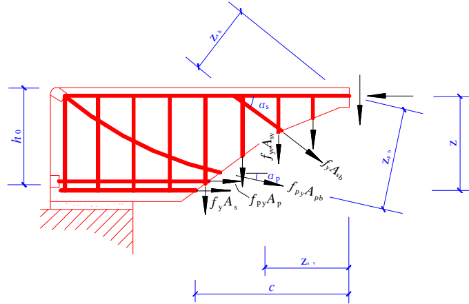
图 7.5.9 受弯构件斜截面受弯承载力计算
