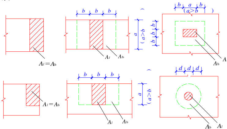
图 7.8.2 局部受压的计算底面积
