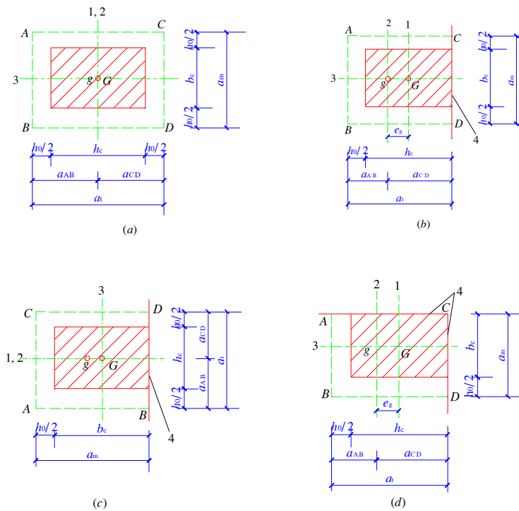
图 G.0.1 矩形柱及受冲切承载力计算的几何参数
