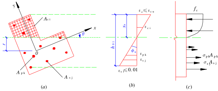
图 F.0.1 任意截面构件正截面承载力计算
