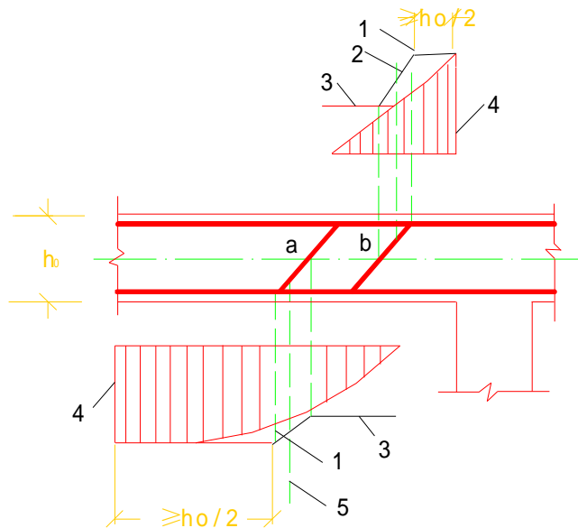
图 10.2.8 弯起钢筋弯起点与弯矩图的关系
