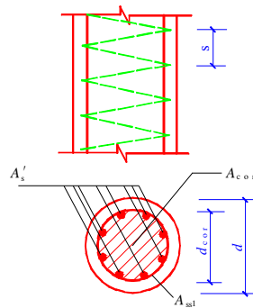
图 7.3.2 配置螺旋式间接钢筋的钢筋混凝土轴心受压构件
