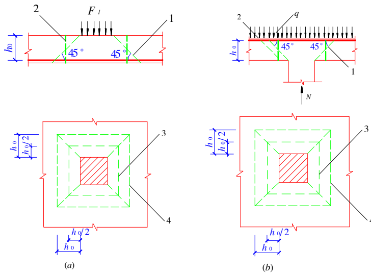
图 7.7.1 板受冲切承载力计算
