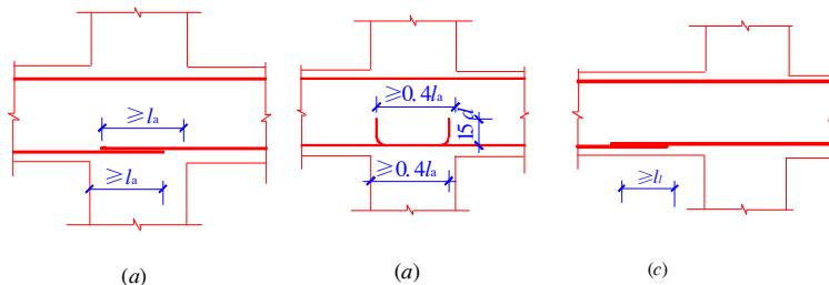
图 10.4.2 梁下部纵向钢筋在中间节点或中间支座范围的锚固与搭接 (a) 节点中的直线锚固；(b) 节点中的弯折锚固；(c) 节点或支座范围外的搭接
