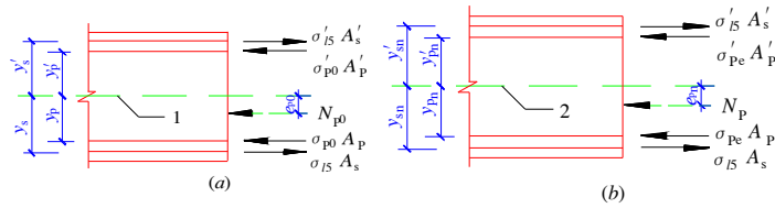
图 6.1.6 预应力钢筋及非预应力钢筋合力位置
