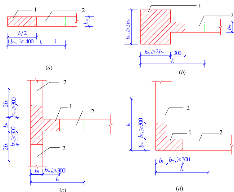
图 11.7.15 剪力墙的约束边缘构件
