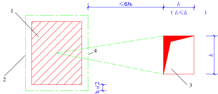
图 7.7.2 邻近孔洞时的临界截面周长
