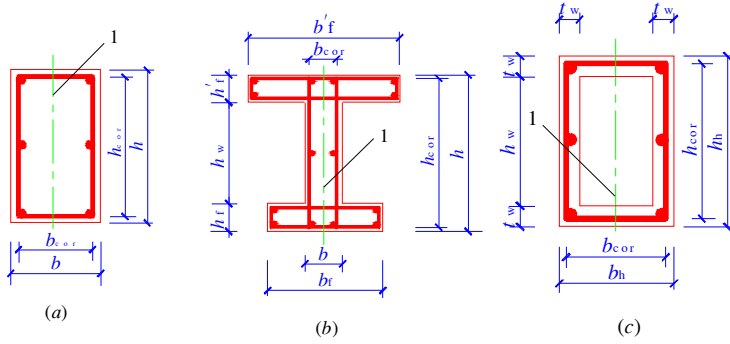
图 7.6.1 受扭构件截面
