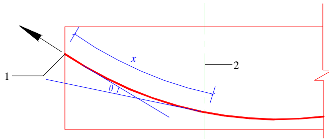
图 6.2.4 预应力摩擦损失计算
