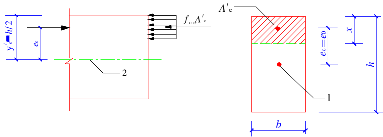
图 A.2.1 矩形截面的素混凝土受压构件受压承载力计算
