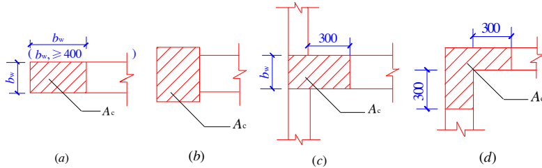
图 11.7.16 剪力墙的构造边缘构件 (a) 暗柱；(b) 端柱；(c) 翼墙；(d) 转角墙
