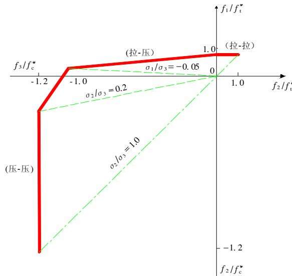
图 C.3.2 混凝土的二轴强度包络图
