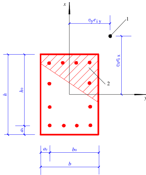
图 7.3.14 双向偏心受压构件截面 1—轴向压力作用点；2—受压区
