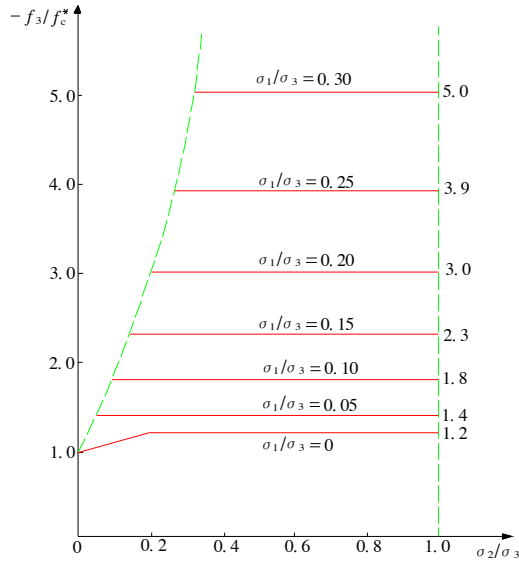
图 C.3.3 混凝土的三轴抗压强度
