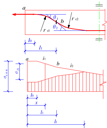
图 D.0.2 两条圆弧形曲线组成的预应力钢筋的预应力损失 \sigma_{\text{fl}}
