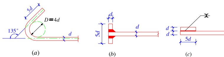
图 9.3.2 钢筋机械锚固的形式及构造要求 (a) 末端带 135°弯钩；(b) 末端与钢板穿孔塞焊；(c) 末端与短钢筋双面贴焊
