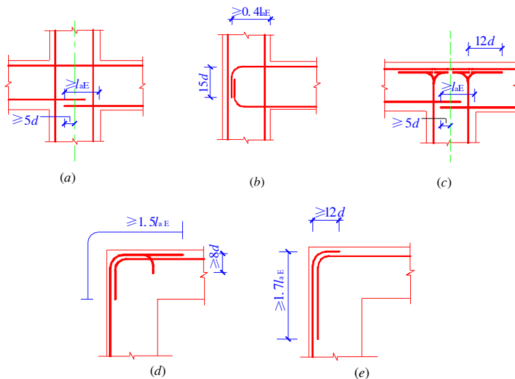
图 11.6.7 框架梁和框架柱的纵向受力
