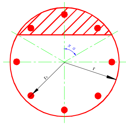
图 7.3.8 沿周边均匀配筋的圆形截面
