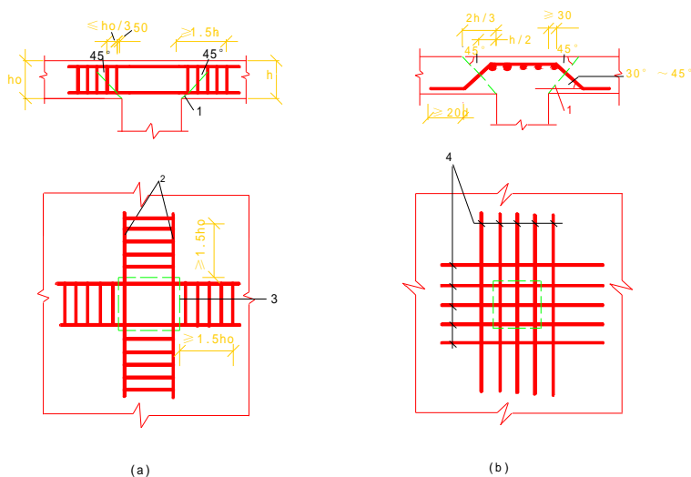
图 10.1.10 板中抗冲切钢筋布置
