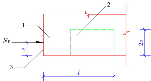
图 9.6.9 防止沿孔道劈裂的配筋范围
