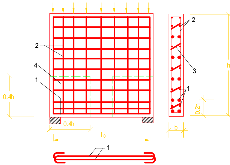
图 10.7.9-1 单跨深梁的钢筋配置
