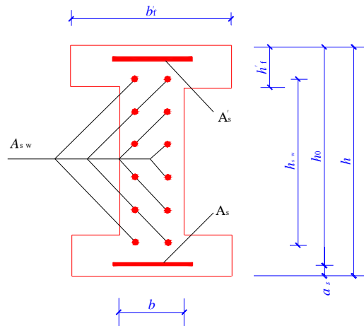
图 7.3.6 沿截面腹部均匀配筋的 I 形截面
