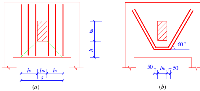
图 10.7.12 深梁承受集中荷载作用时的附加吊筋
