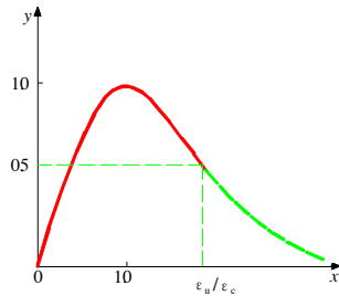
图 C.2.1 单轴受压的应力-应变曲线
