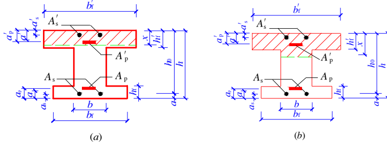
图 7.2.2 I 形截面受弯构件受压区高度位置
