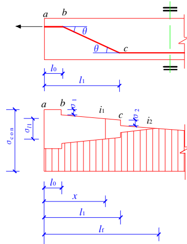
图 D.0.3 折线形预应力钢筋的 预应力损失 \sigma_u
