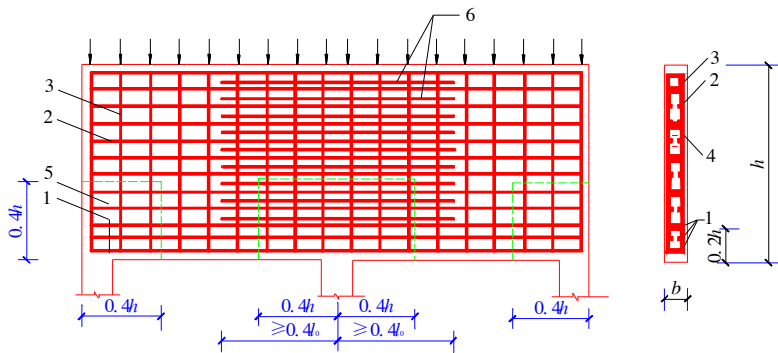
图 10.7.9-2 连续深梁的钢筋配置
