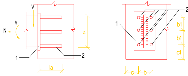
图 10.9.1 由锚板和直锚筋组成的预埋件 1—锚板；2—直锚筋
