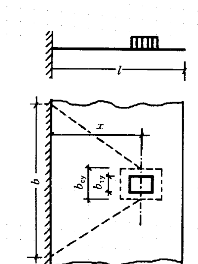
图 B.0.5-4 悬臂用板上局部荷载的有效分布宽度
