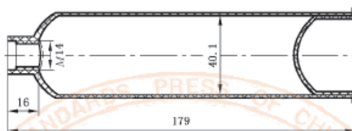
图 1 挤出性试验用挤胶筒
