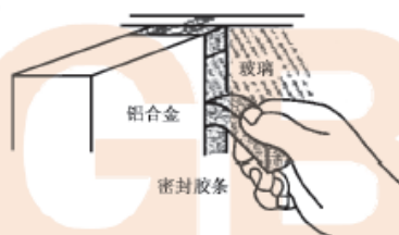
图 D.1 90°角拉扯密封胶
