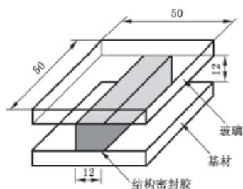
图 2 拉伸粘结试件
