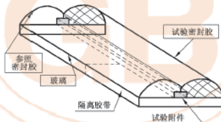
图 A.3 附件相容性试验的试件形式
