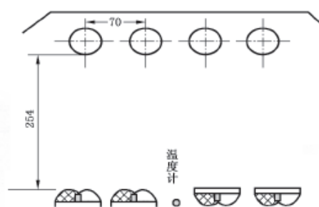
图 A.2 紫外线曝晒形式
