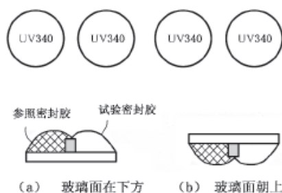
图 A.1 光照试件的放置
