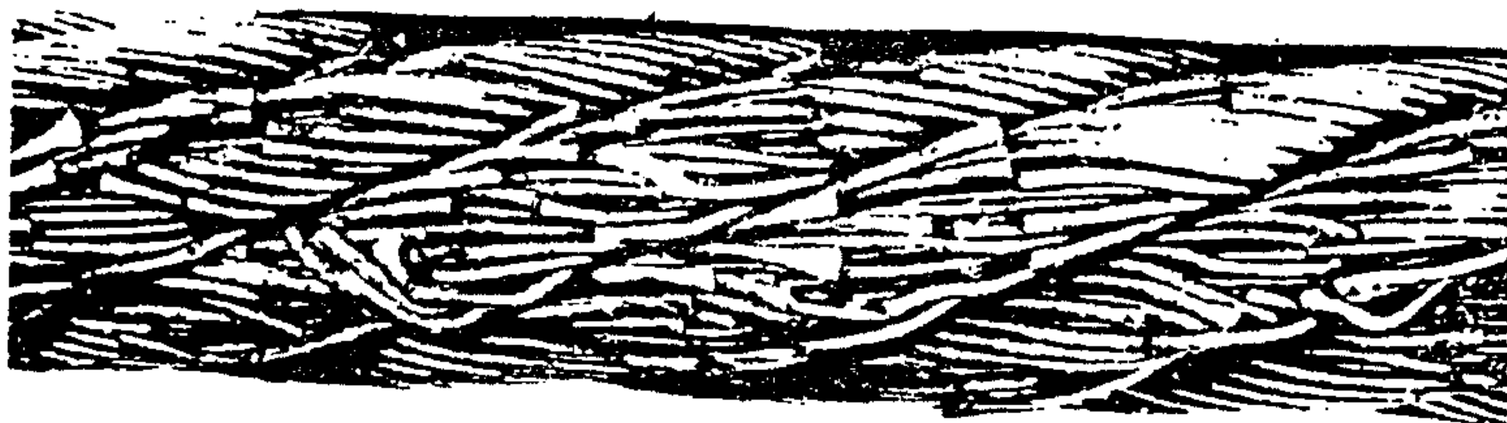
图 E.2 交互捻钢丝绳大量断丝伴随着严重的磨损——应立即报废
