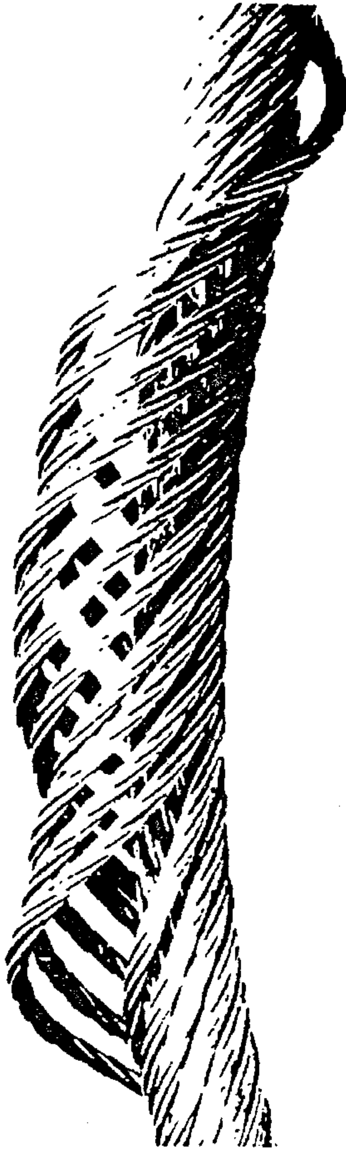
图 E.9 多股绳的笼状(鸟笼形)畸变——应立即报废
