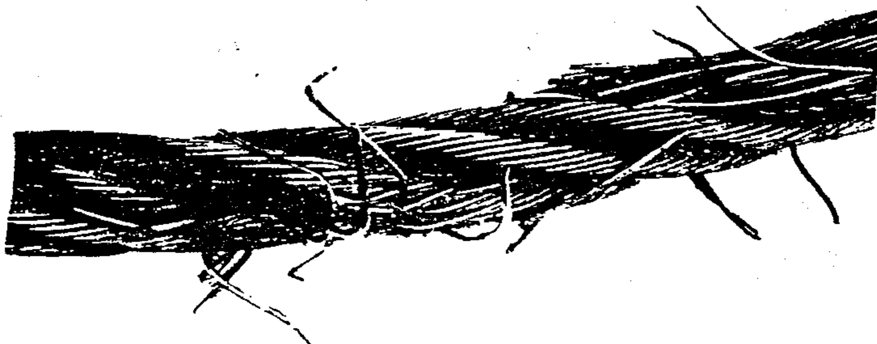
图 E.21 当钢丝绳已跳出滑轮绳槽并被楔住的典型示例：已经形成“部分被压扁”形式的变形并有局部磨损和许多断丝——应立即报废
