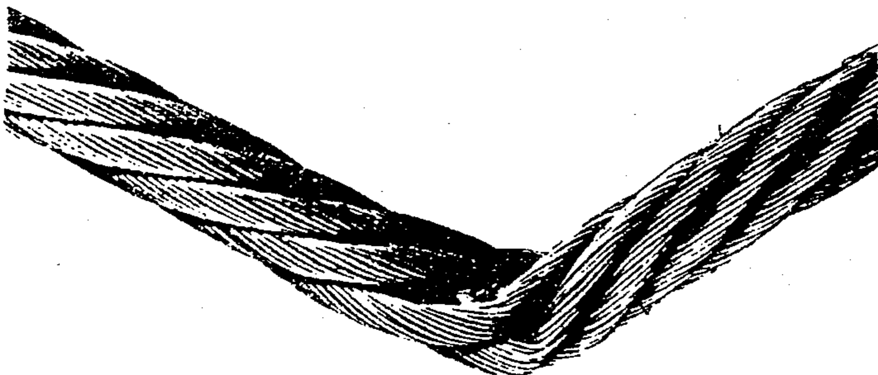
图 E.20 严重弯折之一例——应报废
