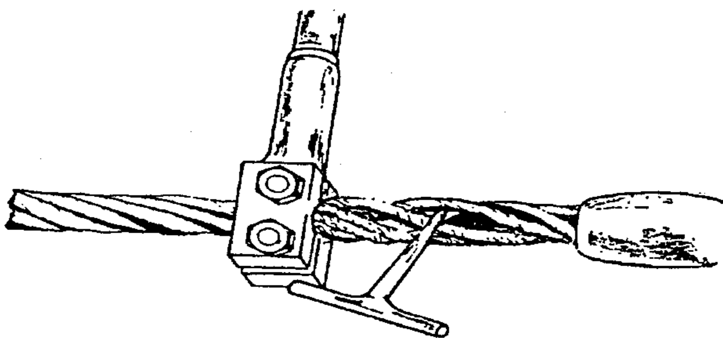
图 D.2 对靠近接头的钢丝绳尾部作内部检验(张力为零)
