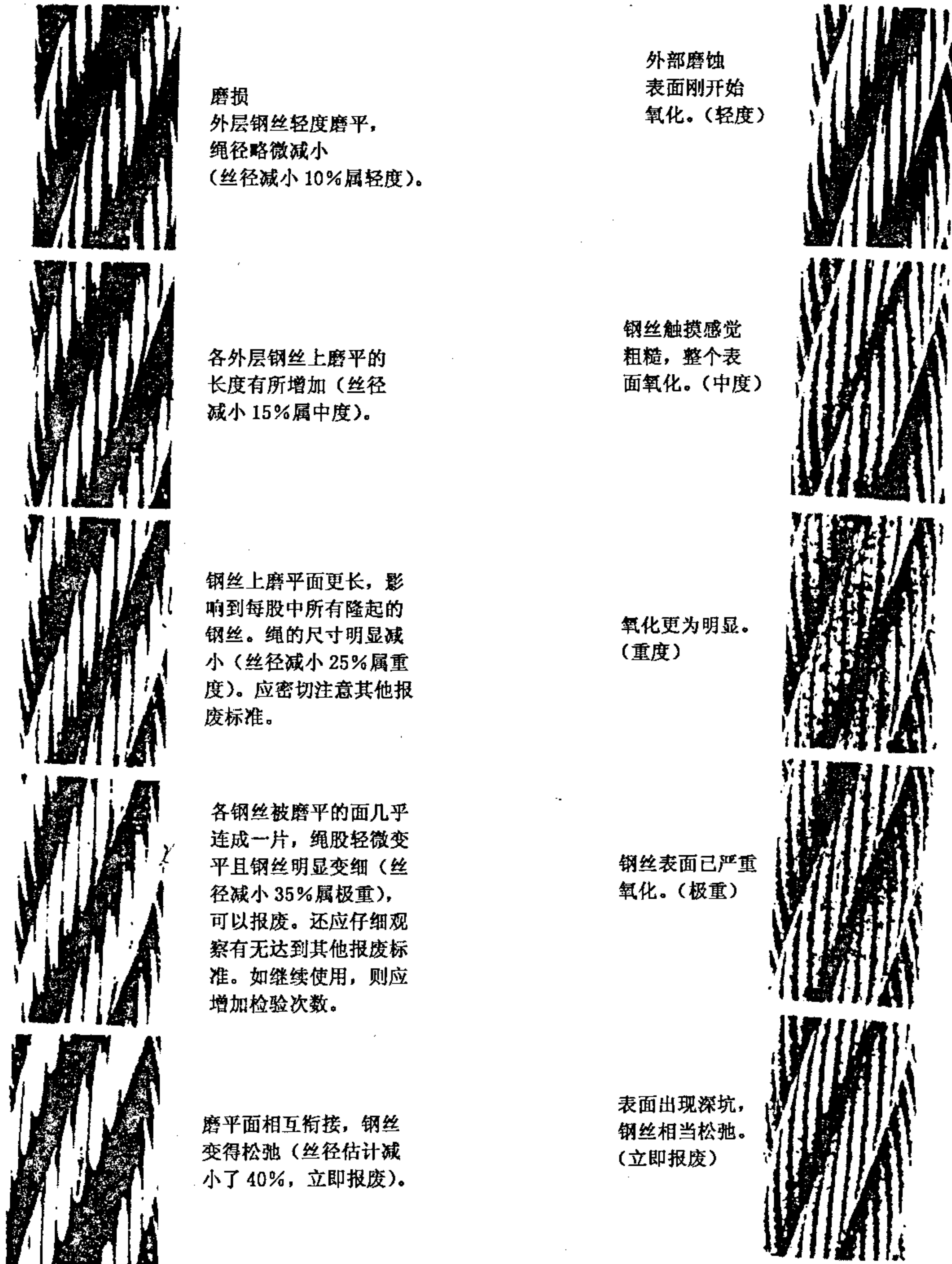
图 E.4 交互捻钢丝绳的磨损和外部腐蚀的发展过程举例
