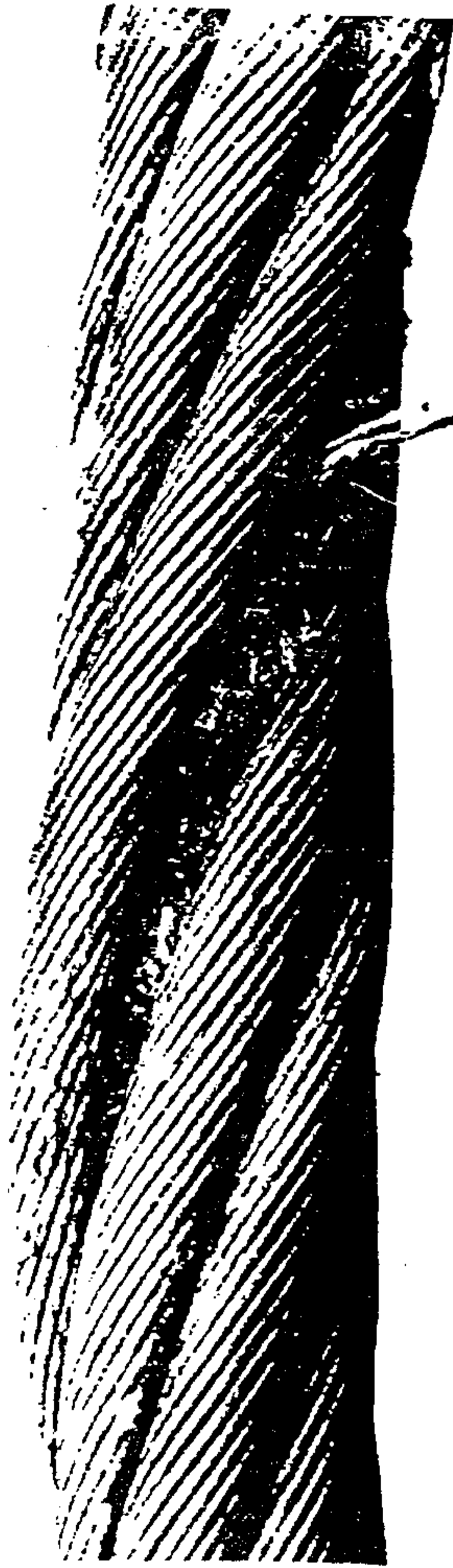
图 E. 14 钢丝绳直径的局部增大:是由于纤维芯变质在外层股间突出而引起——应报废
