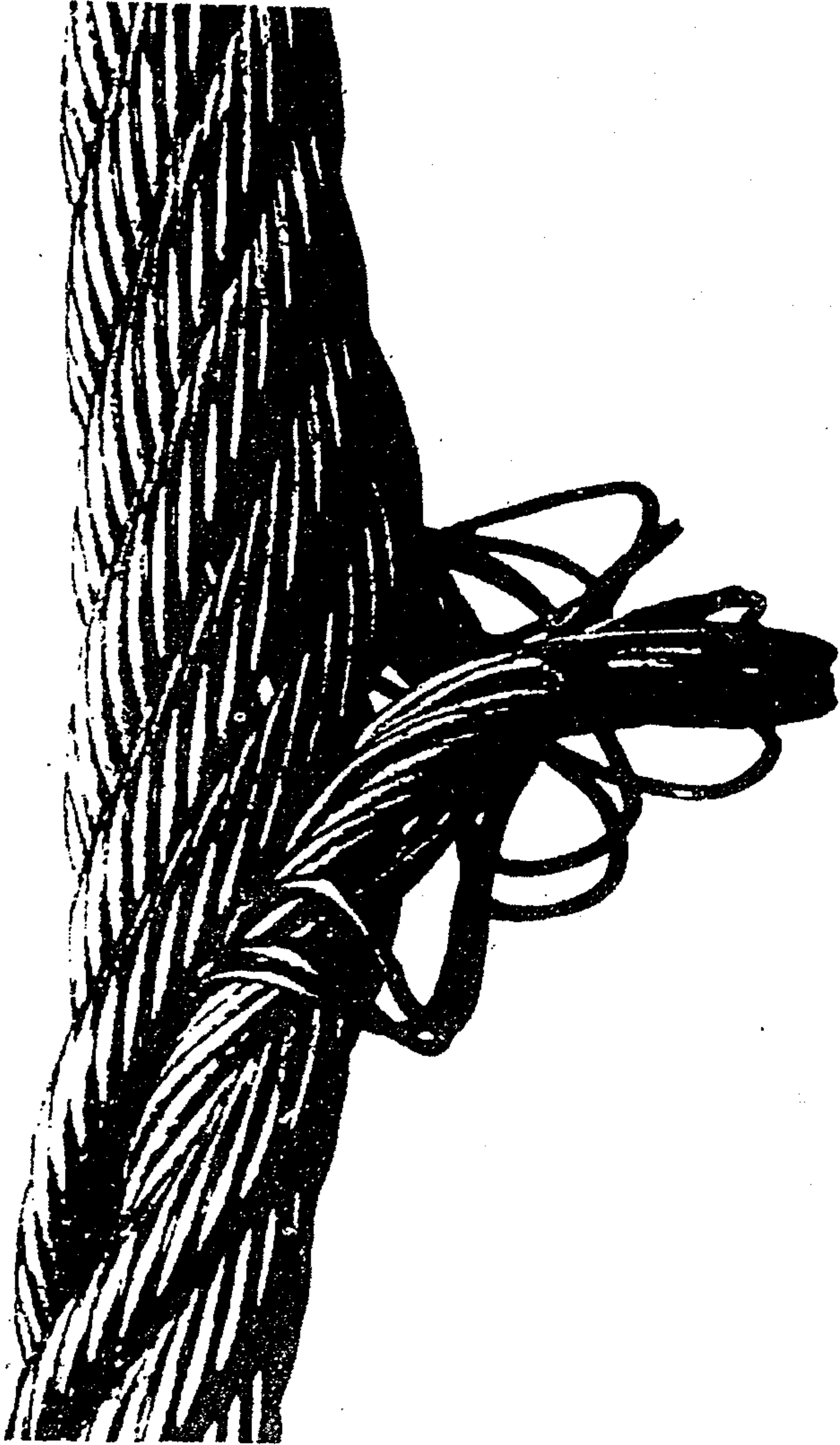
图 E.10 钢芯挤出,通常伴随着邻近位置的笼状畸变——应立即报废
