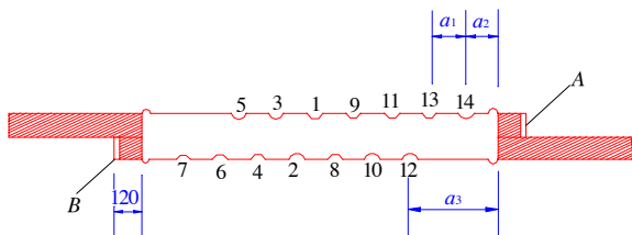
LGJ-35 钢芯铝绞线
