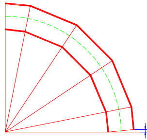
图 5.2.5-2 焊制弯管 端面垂直偏差
