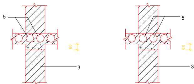
(b)新增设横墙与预制空心楼面的连接
