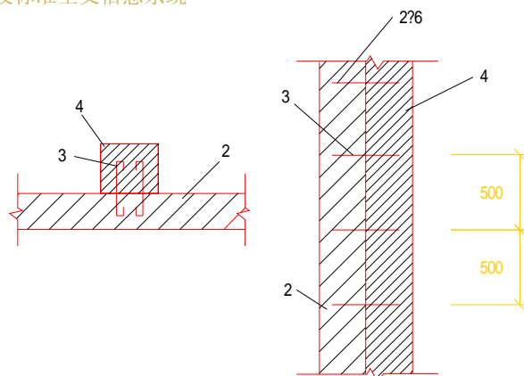
(a) 砖壁柱与原墙连接
