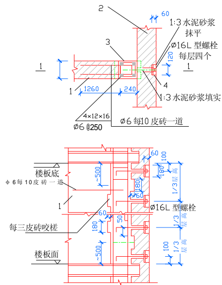
图 5.2.7.4 新增设墙体与原墙体连接构造图 1—新增设墙;2—原墙体;3—C20 混凝土横墙砌完后浇筑; 4—钢垫板 180×120×8(mm)
