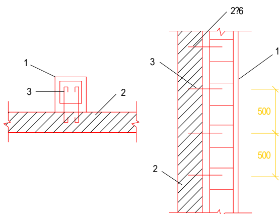
(b) 混凝土柱与原墙连接
