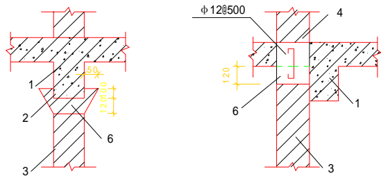
(a)新增设横墙与现浇楼盖的连接
