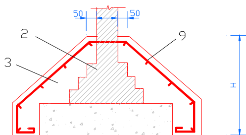
图 4.2.1 壁柱基础及条形基础加大的连接
