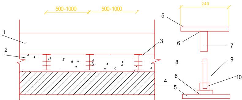
(a)宽支座法卸荷图 (b)旋顶装置意图
