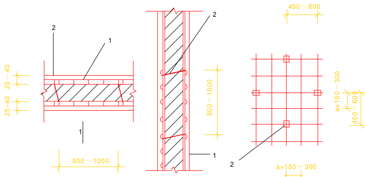
(b) 夹板墙
