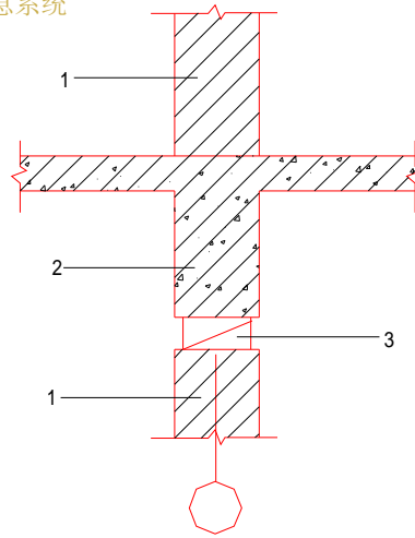
图 4.2.5 新增设墙体顶部与梁的连接 1—新增设墙体；2—钢筋混凝土大梁；3—钢楔间距 500mm
