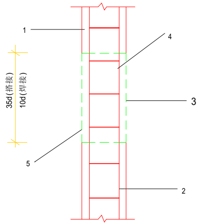
(a) 新旧钢筋混凝土构造柱连接
