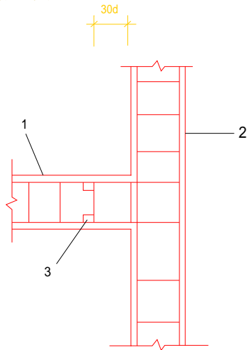
图 5.2.2 新增设墙体圈梁与原墙体圈梁连接
