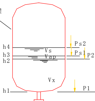
4.3.4—2 隔膜式气压水罐
