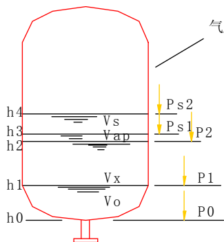
图 4.3.4—1 补气式气压水罐
