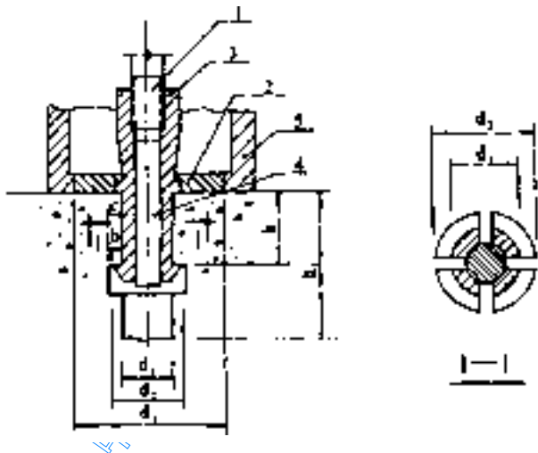
图 3.1.3.1 圆环式拔出试验装置示意图
