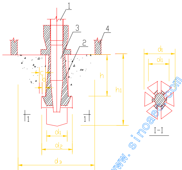
图 3.1.3-2 三点式拔出试验装置示意图
