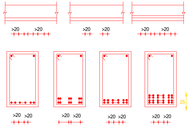
图6.1.3 双钢筋在构件中的排放形式
