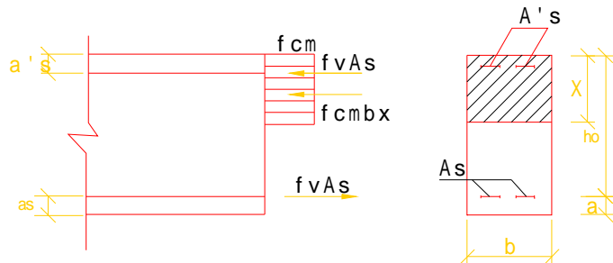
图 4.0.1 矩形截面受弯构件正截面承载力计算
