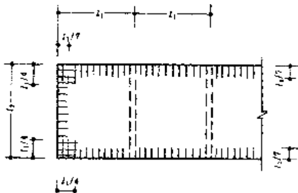
图6.2.7 板嵌固在承重砖墙内时板边构造钢筋配筋
