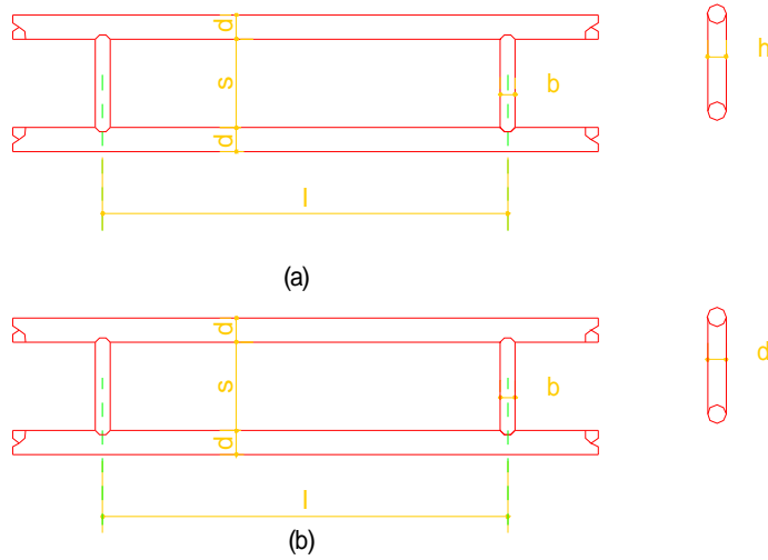
图 2.2.3 双钢筋纵筋与横筋的组成 (a) 平焊矩形横筋的双钢筋； (b) 平焊圆横筋的双钢筋
