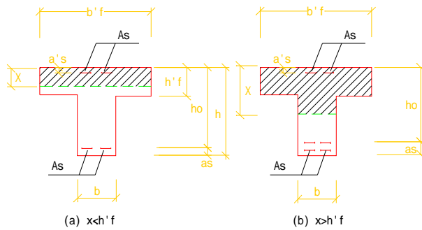
图4.0.2 T形截面受弯构件受压区高度位置
