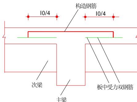
图6.2.5 板中与梁肋垂直的构造钢筋配筋
