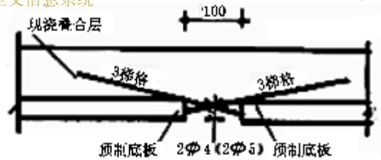
图6.2.8-1 底板拼缝构造
