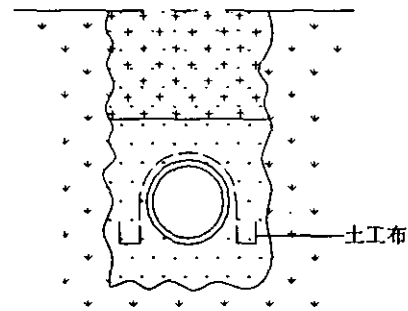
图 2 防管道上浮的土工布包覆方法
