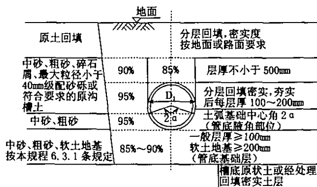
图 8.2.5 沟槽回填土要求
