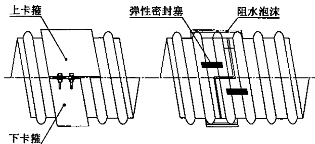
图 6.4.4-4 卡箍连接
