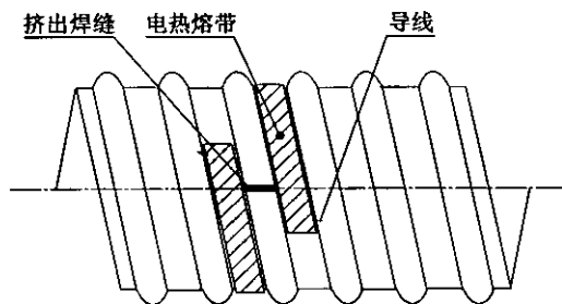
图 6.4.4-2 电熔带连接
