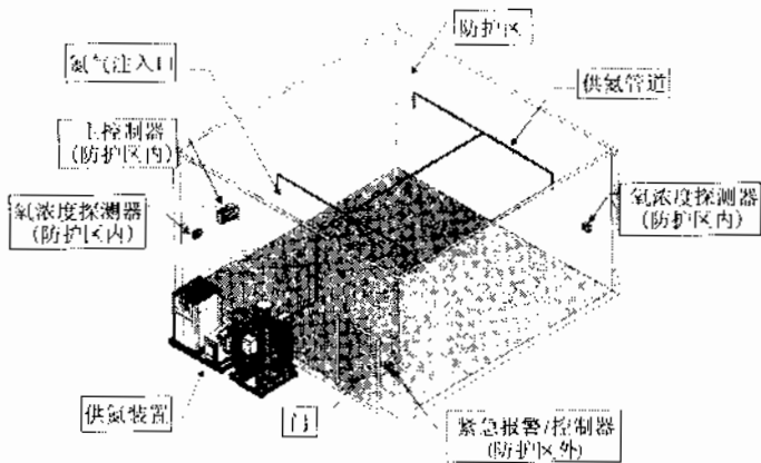
图 C.0.2 有管网系统注氮方式
