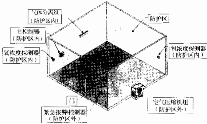
图 C.0.1 无管网系统注氮方式
