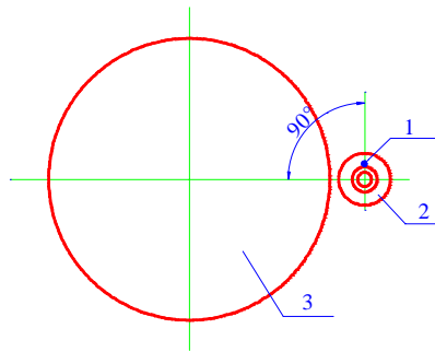
图 5.2.5 烟雾产生器安装位置 1—导火索头盖接头;2—烟雾产生器;3—储罐
