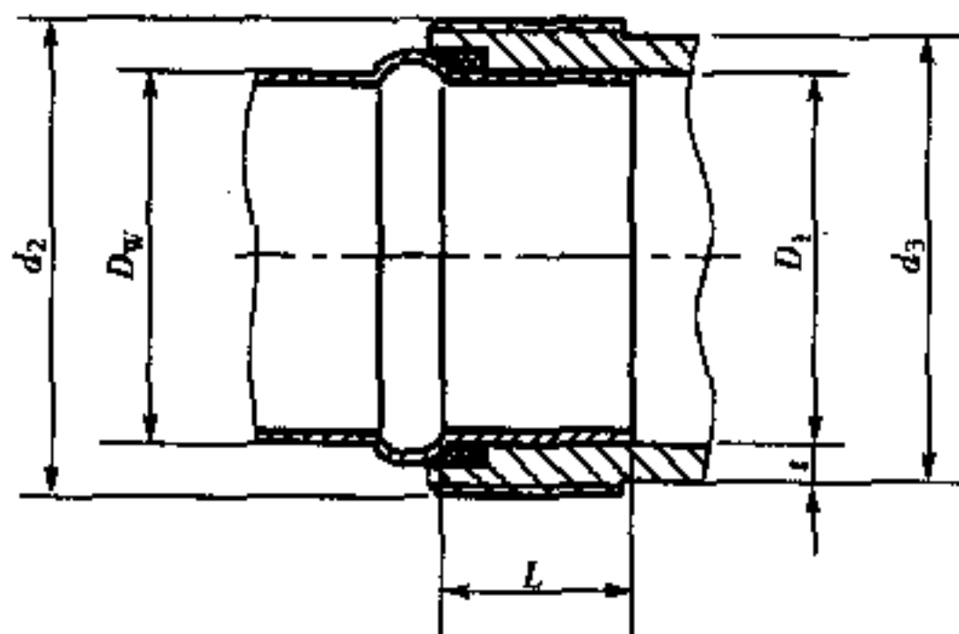
图 C.0.1 不锈钢压缩式管件承口
