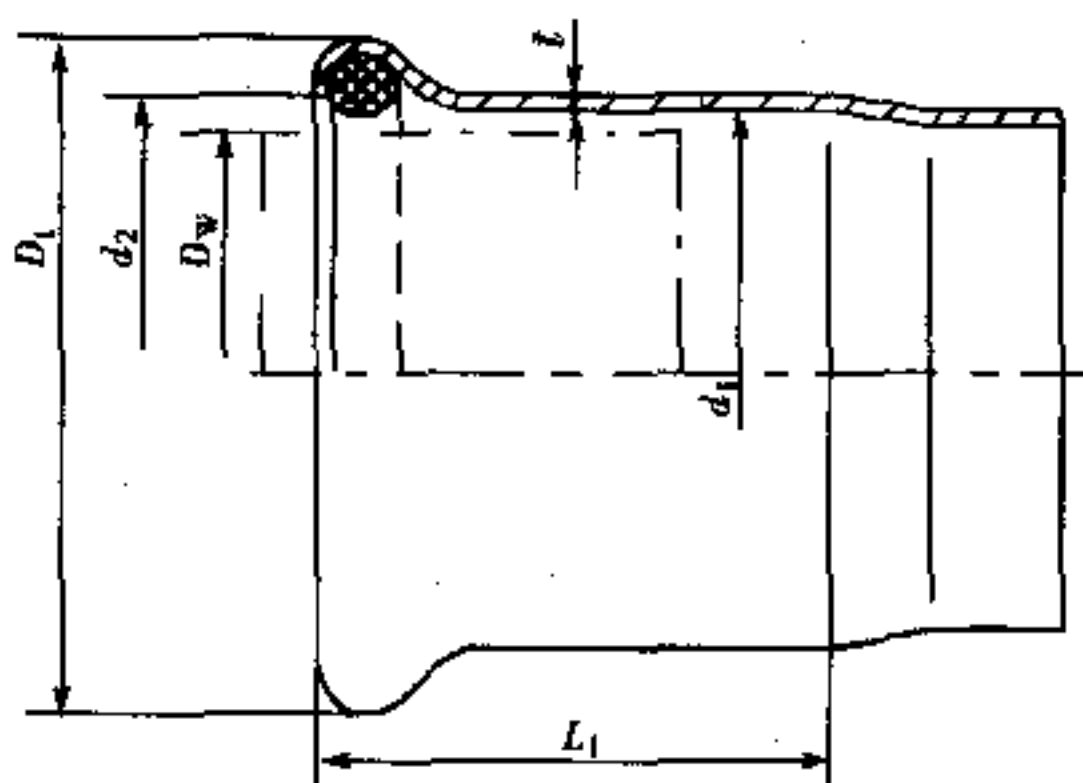
图 B.0.1 不锈钢卡压式管件承口
