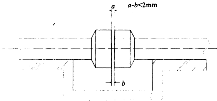
图 6.3.2 法兰连接
