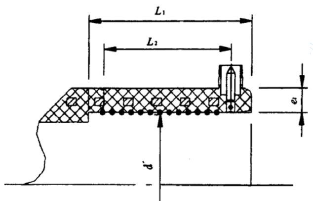
图 3.3.2 钢板孔网骨架聚乙烯复合电热熔管件示意图
