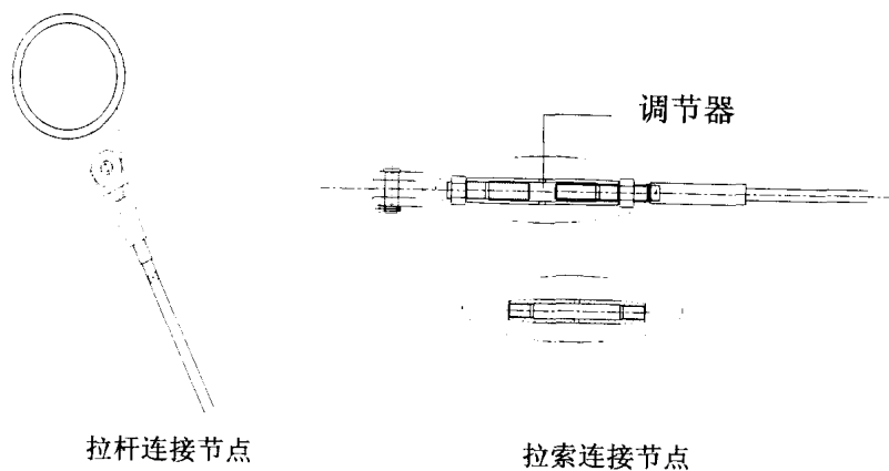
图 5.7.5 拉杆、拉索连接节点
