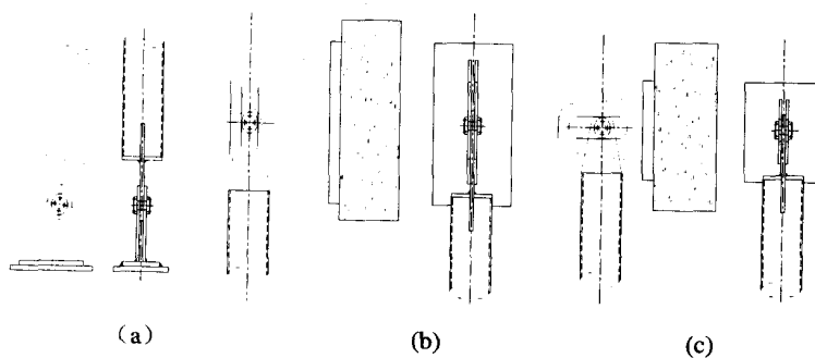
图 5.7.4 销钉连接
