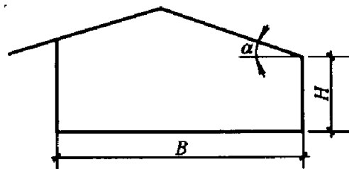
图 A.0.2-3 挑檐的风荷载体型系数分区
