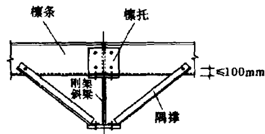
图 7.2.14 隔撑的连接
