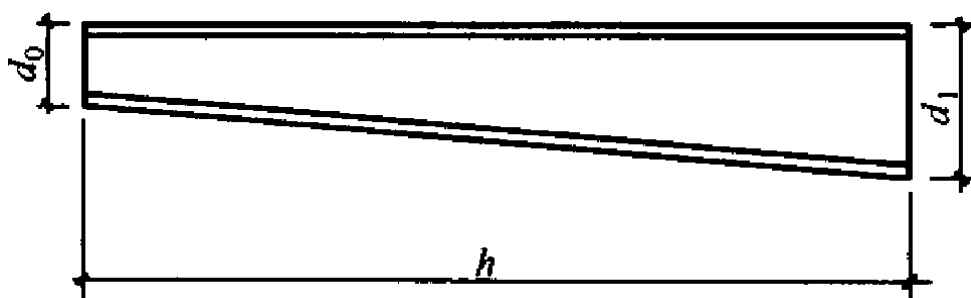
图 6.1.3-3 变截面构件的楔率
