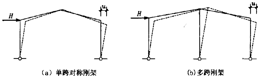
图 6.1.3-2 一阶分析时的柱顶侧移
