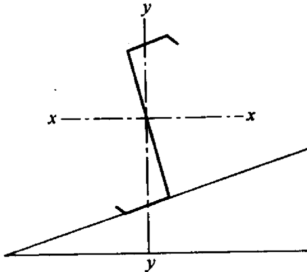
图 6.3.7 檩条的主轴
