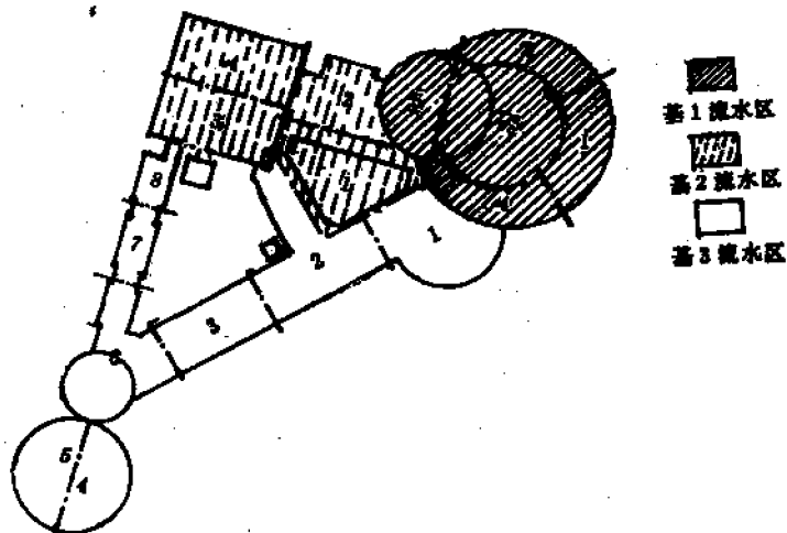
图 2.1.8(2) 基础分区分段示意图
