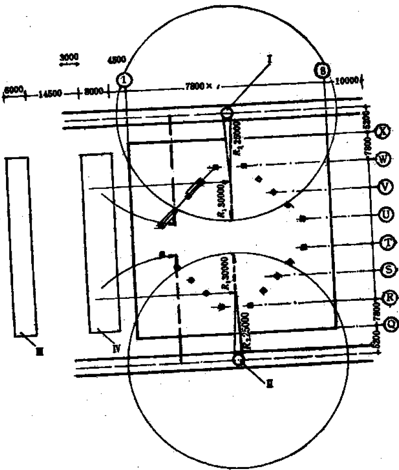
图 2.1.8(4) 600 座小型国际会议厅大跨度吊装平面示意 I—TQ60/80 塔吊 1#; II—TQ60/80 塔吊 3#; III—钢结构拼装台 6m×50m; IV—钢结构临时堆场 8m×50m
