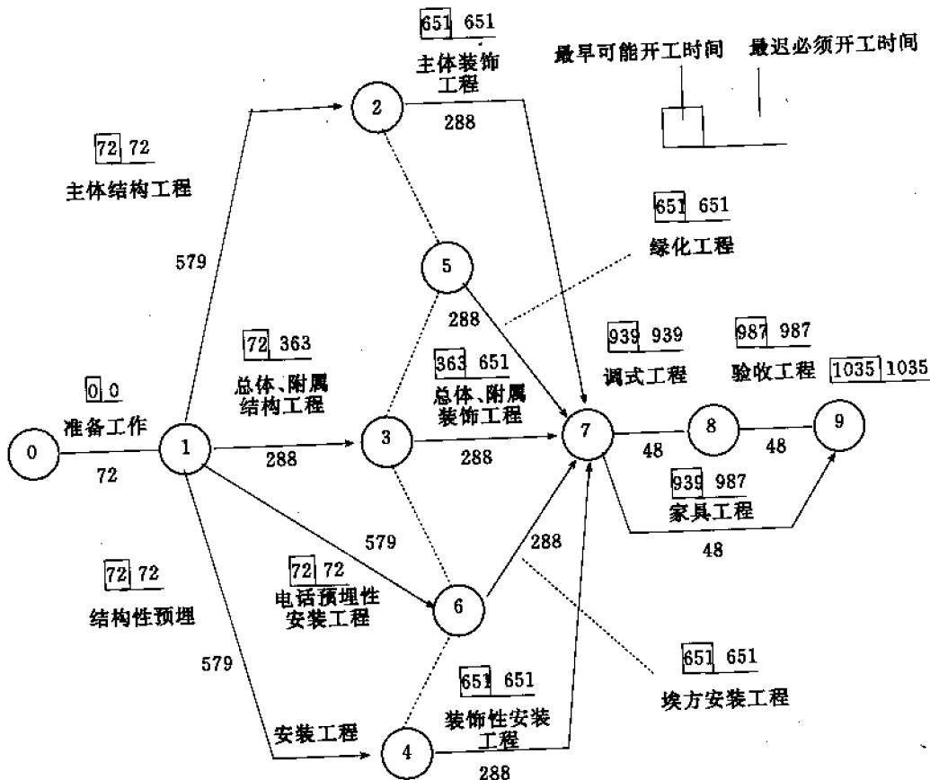
图2.1.8(6) 开罗国际会议中心施工总网络图(一级网络)
