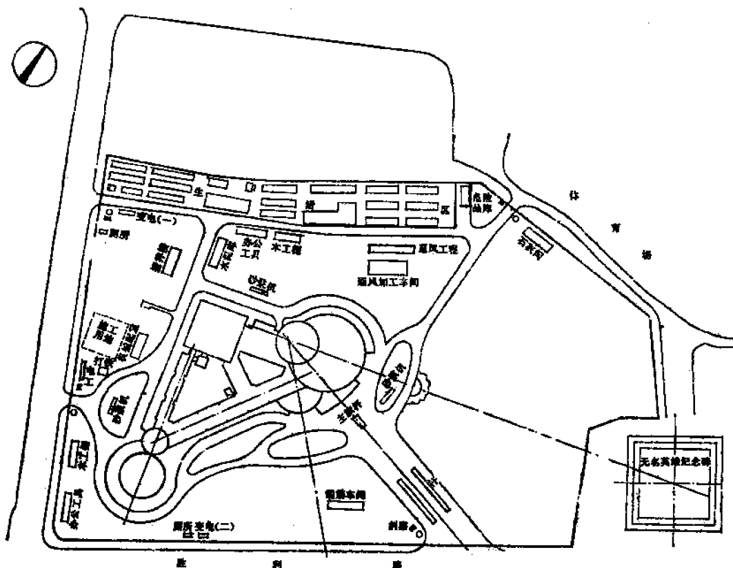
图 2.1.8(7) 施工准备阶段施工总平面图
