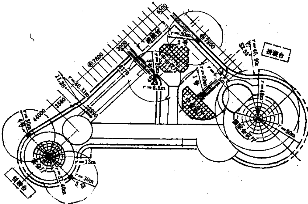
图 2.1.8(1)为国际会议中心塔吊布设总图。
