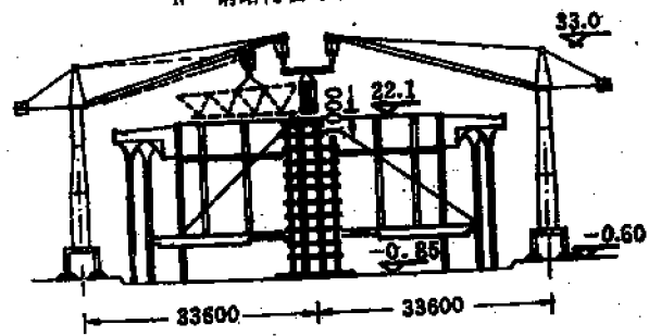
图 2.1.8(5) 宴会厅空间网架立面吊装示意
