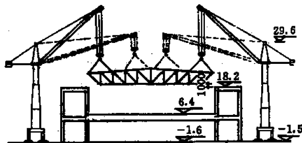
图 2.1.8(3) 600座小型国际会议厅大跨度桁架吊装立面示意图
