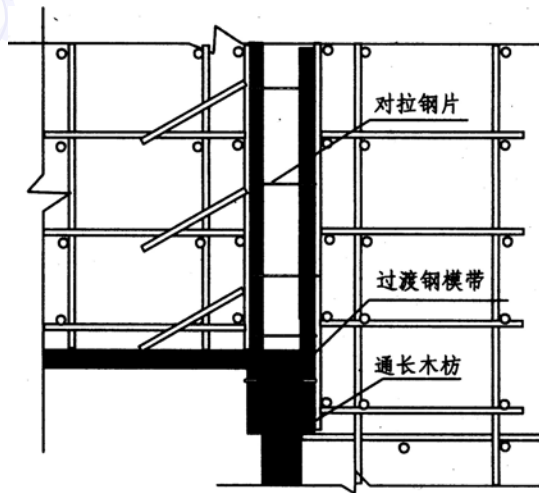
图 7-7 外剪力墙楼面板接头支模示意图
