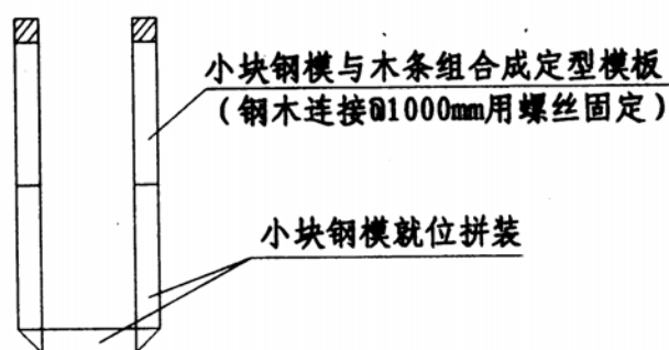
图 7-8 木模拼嵌示意图
