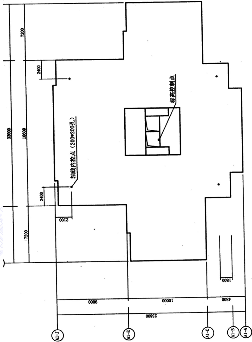
A1型房轴线标高控制图
