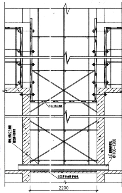
图 7-6 电梯井筒模板及支撑安装图
