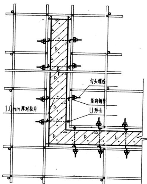
图 7-2 对拉片示意图
