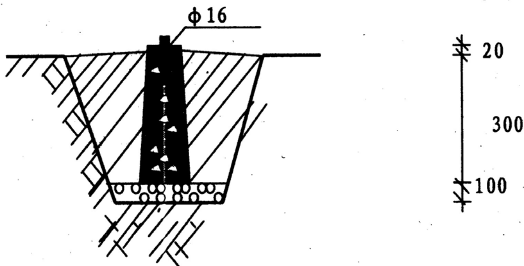
图 6-1 控制桩埋设方法
