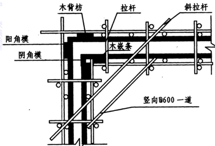
图 7-5 角模支模示意图
