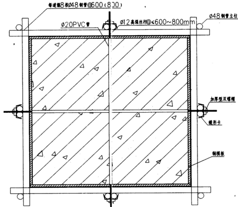
图 7-1 800mm 以上断面方柱支模大样图
