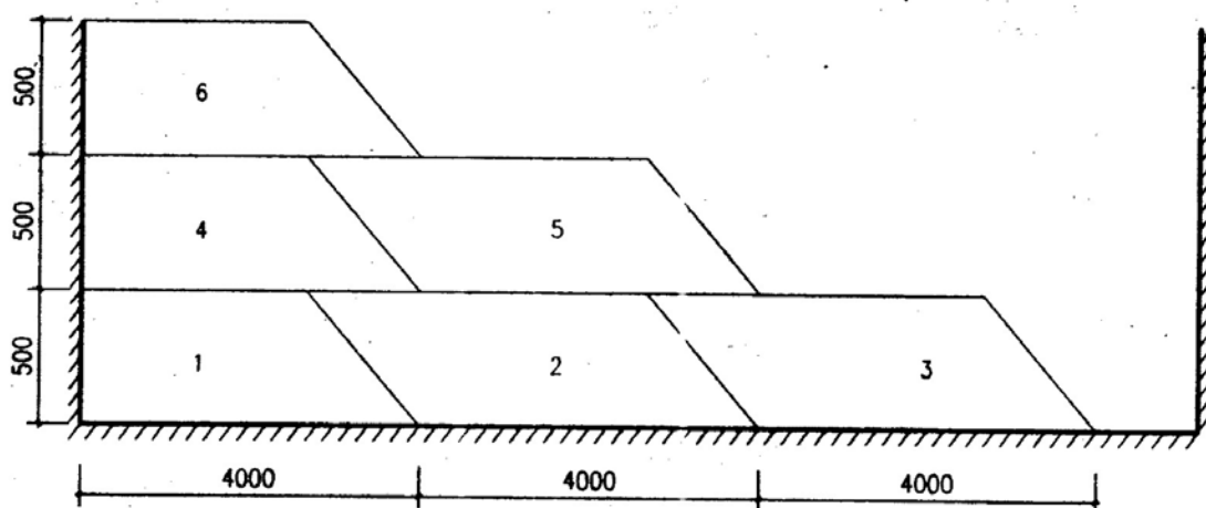
图 6-4 推进浇筑混凝土示意图
