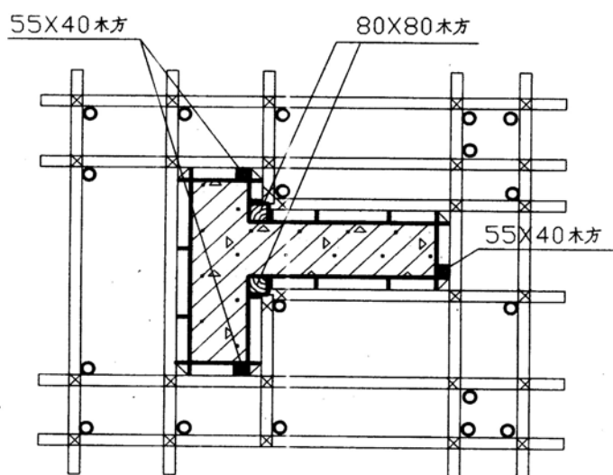
图 7-3 薄壁柱模板支撑详图
