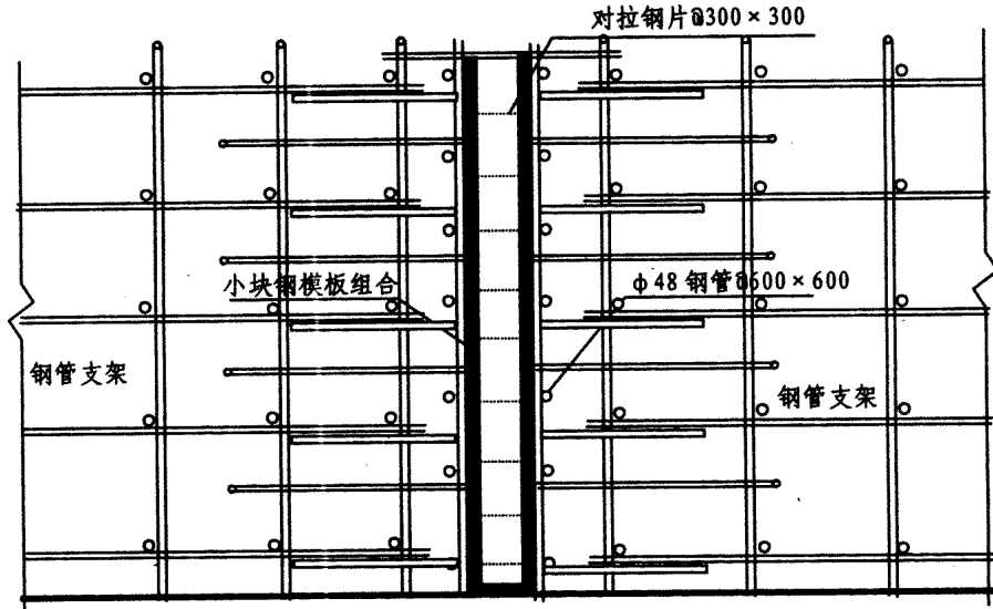
图 7-4 剪力墙支模示意图
