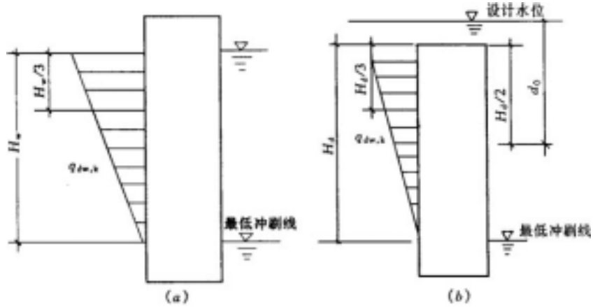
图 4.3.4 作用在取水头部上的流水压力图
